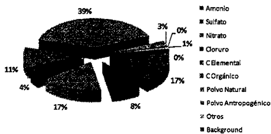
Componentes PM 2.5 2005
