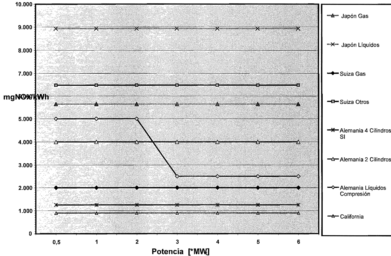
Gráfico N° 11 Límites Internacionales de Emisión de NOx para Motores
