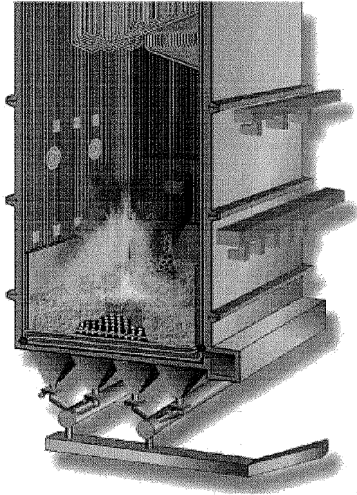
Caldera Lecho Fluidizado Burbujeante
