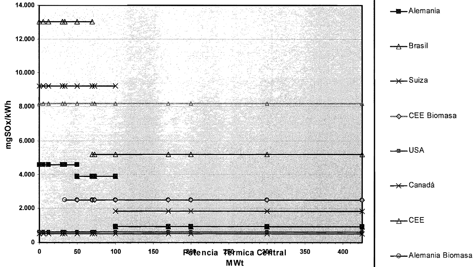
Gráfico N° 4 Límites Internacionales de SO 2 para Turbinas a Vapor con Combustibles Sólidos
