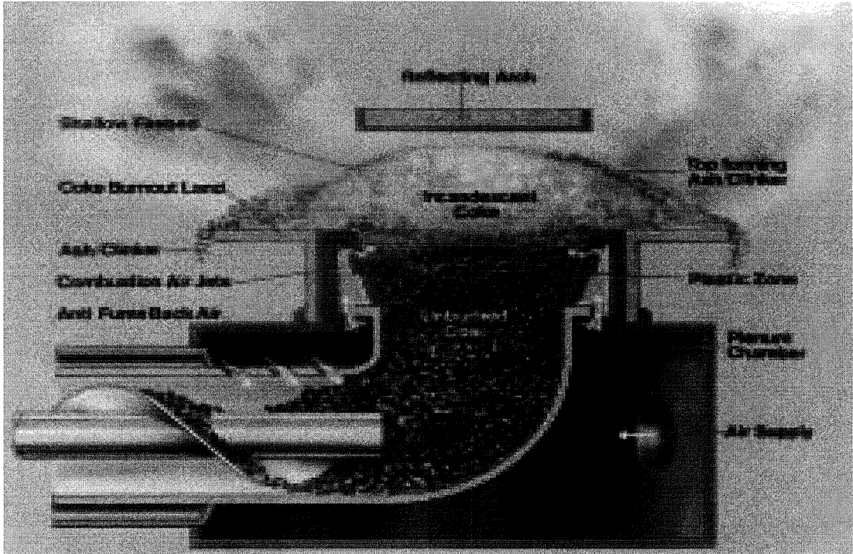
Figura N° 2: Parrilla de Alimentación Inferior Fuente: DTI Fuel Cleaner Fossil Fuel Programme. UK
