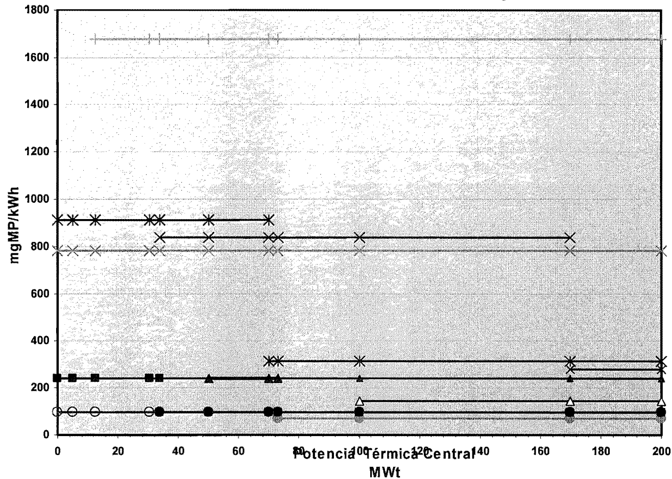
Gráfico N° 2 Límites Internacionales de Emisiones MP para Turbinas a Vapor con Combustibles Líquidos
