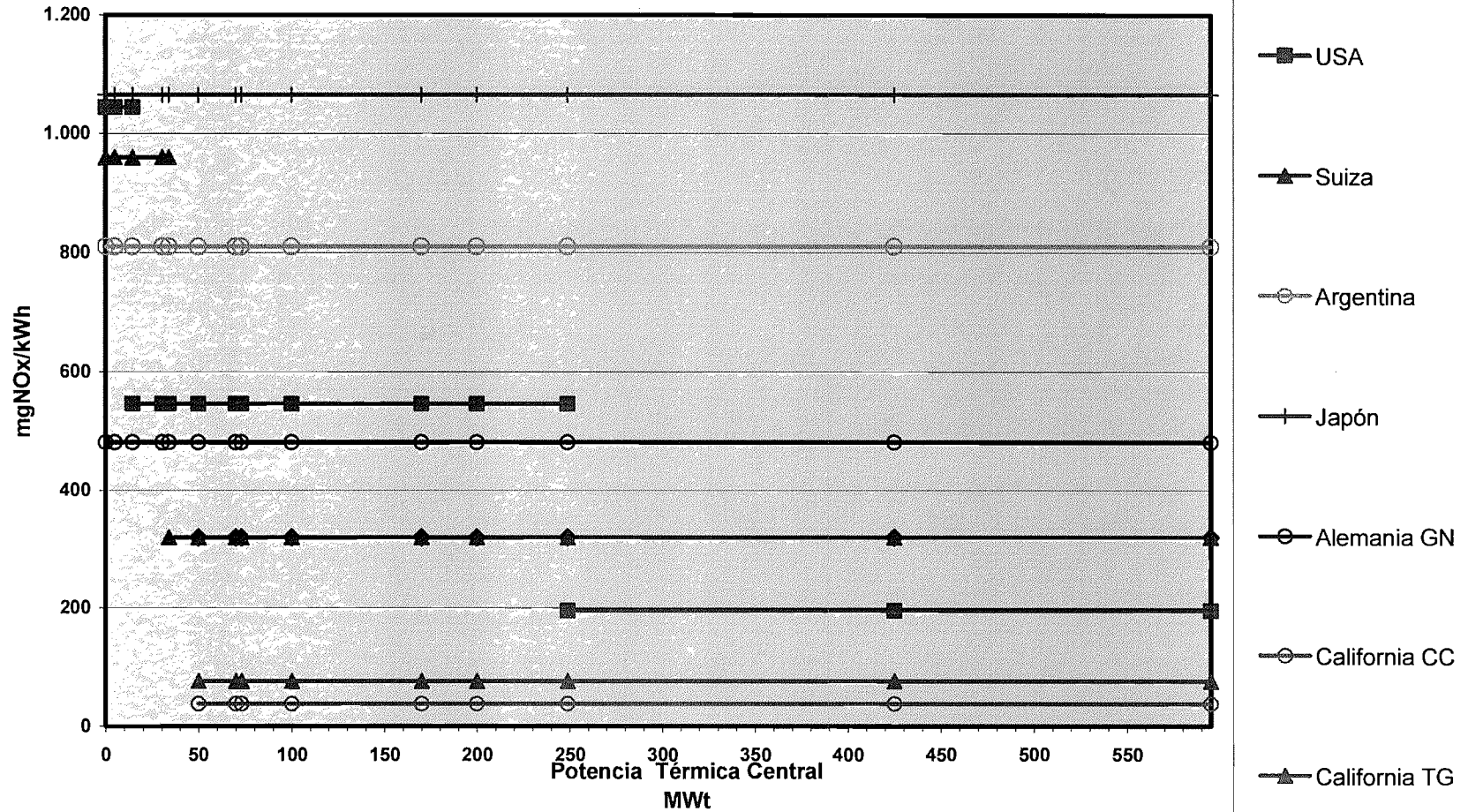
Gráfico N° 10 Límites Internacionales de NOx para TG y Ciclo Combinado con Combustibles Gaseosos
