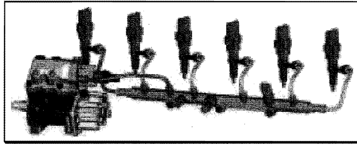
Figura N° 26: Sistema Common-Rail.
