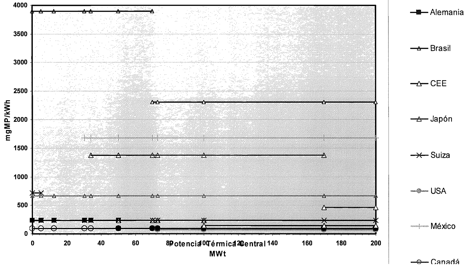
Gráfico N° 1 Límites Internacionales de Emisiones MP para Turbinas a Vapor con Combustibles Sólidos
