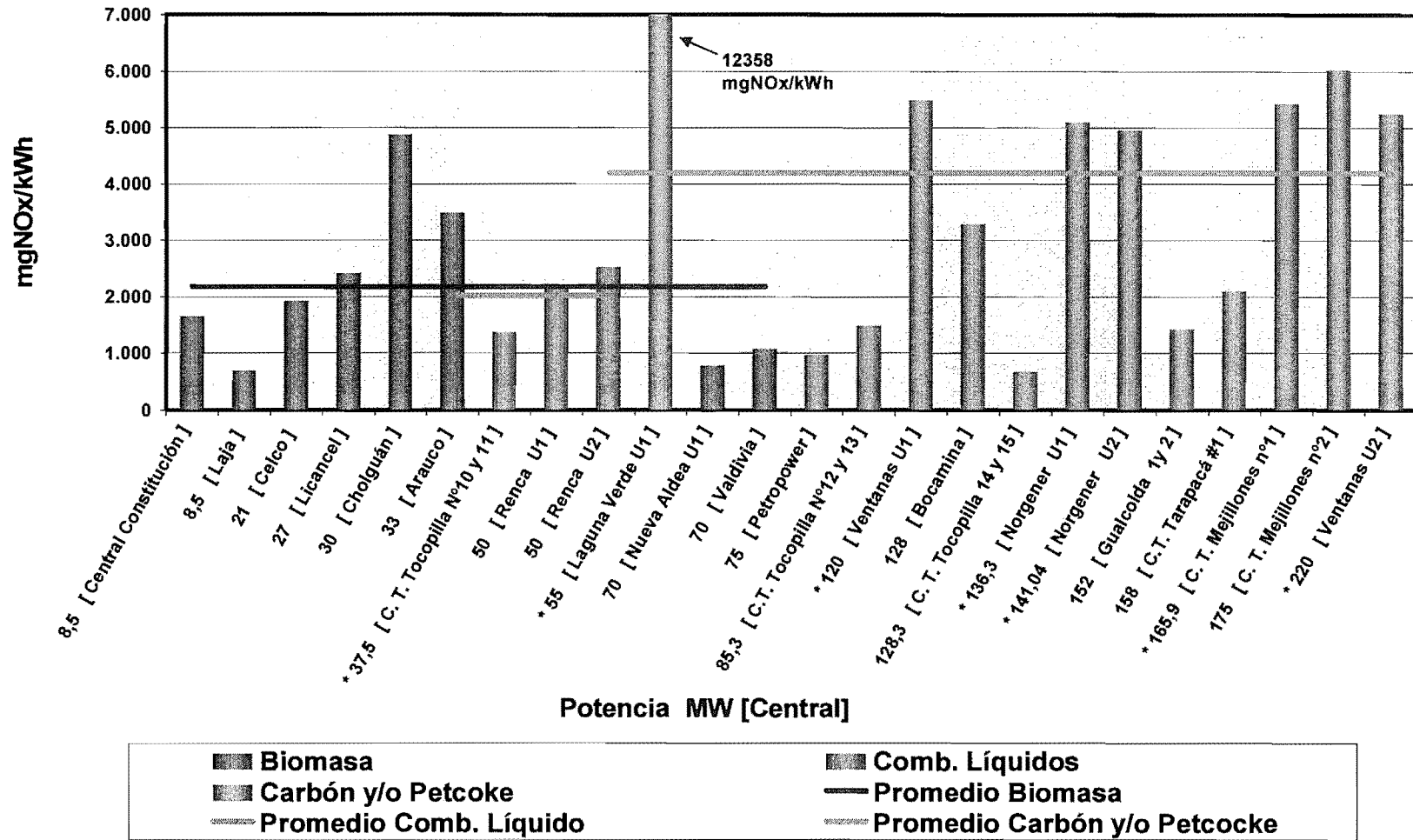
Gráfico N° 25 Emisiones NOx de Centrales con Turbina a Vapor según Potencia Instalada
