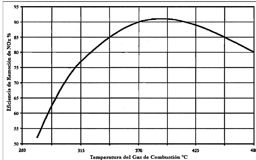
Figura N° 20: Eficiencia de Remoción de NO x , como función de la Temperatura de los Gases de Combustión para un catalizador típico de óxidos metálicos.
