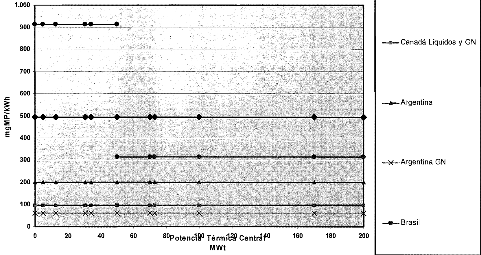
Gráfico N° 3 Límites Internacionales de Emisiones de MP para Turbinas a Gas y Ciclo Combinado
