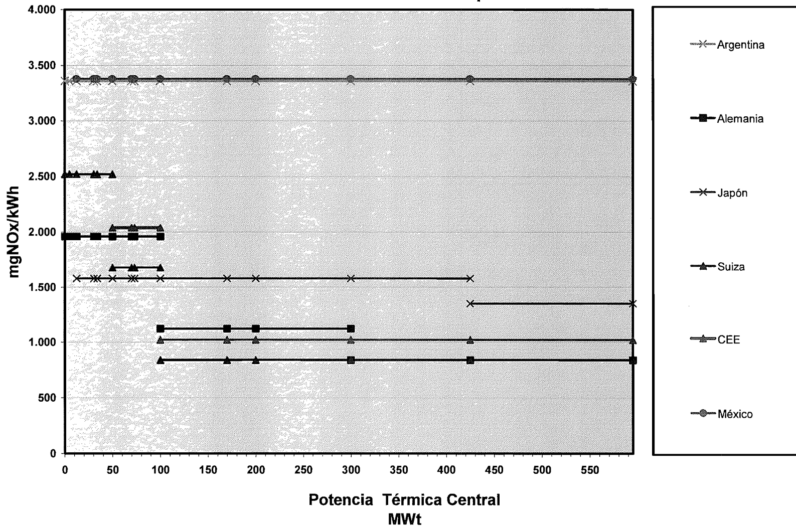
Gráfico N° 8 Límites Internacionales de NOx para Turbinas a Vapor con Combustibles Líquidos
