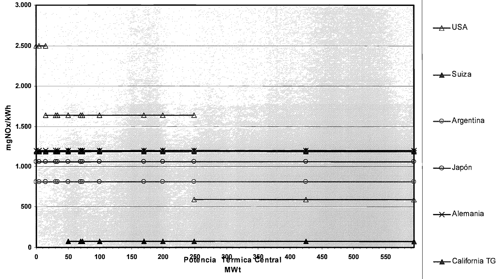
Gráfico N° 9 Límites Internacionales de NOx para TG y Ciclo Combinado con Combustibles Líquidos
