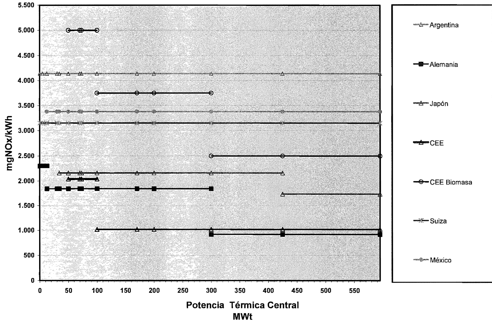
Gráfico N° 7 Límites Internacionales de NOx para Turbinas a Vapor con Combustibles Sólidos
