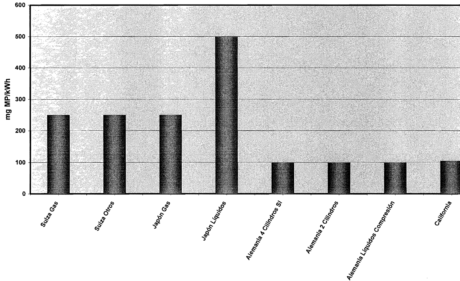
Gráfico N° 12 Límites Internacionales de Emisión de MP para Motores
