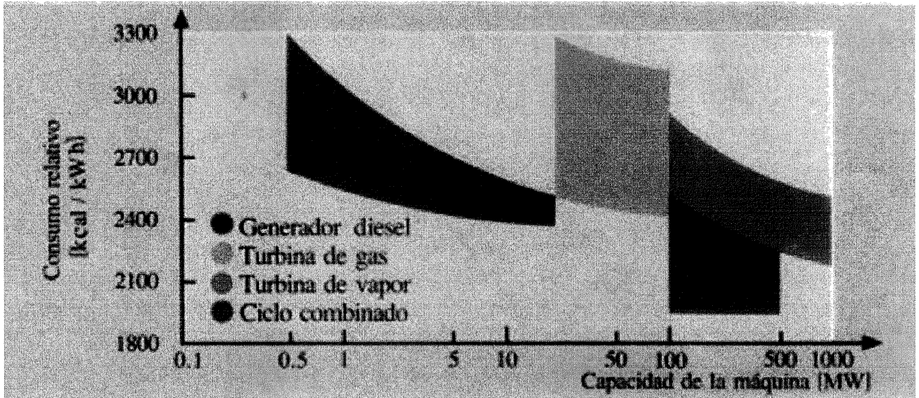
Figura N° 5 : Comparación de Consumos Relativos de Combustible en Centrales Térmicas
