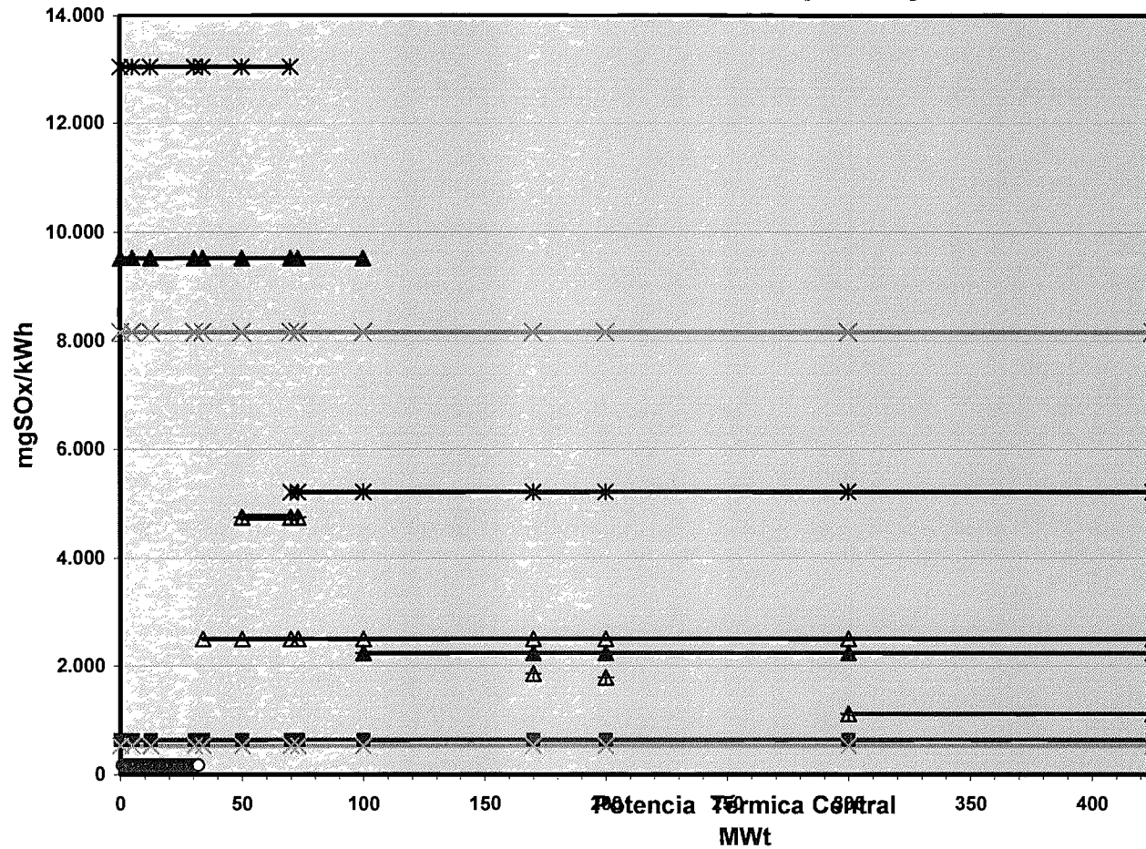
Gráfico N° 5 Límites Internacionales de SO 2 para Turbinas a Vapor con Combustibles Líquidos y Gaseosos
