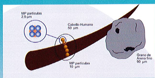
Tamaño de las partículas MP 2,5 y MP 10 (µm =micrómetro)
