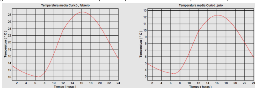
Figura xx: Variación horaria de la temperatura para el mes más cálido y el mes más frío en Curicó.
