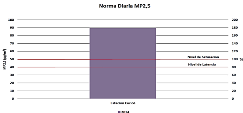
Figura xx: Evaluación Norma 24 Horas de MP2,5, estación Curicó
