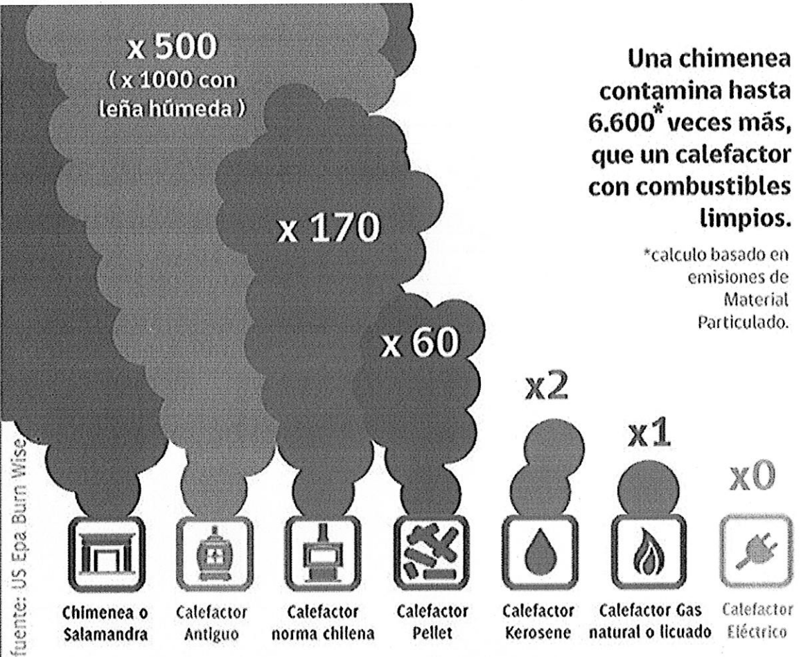
Emisiones de MP comparadas a un calefactor a Gas Licuado
