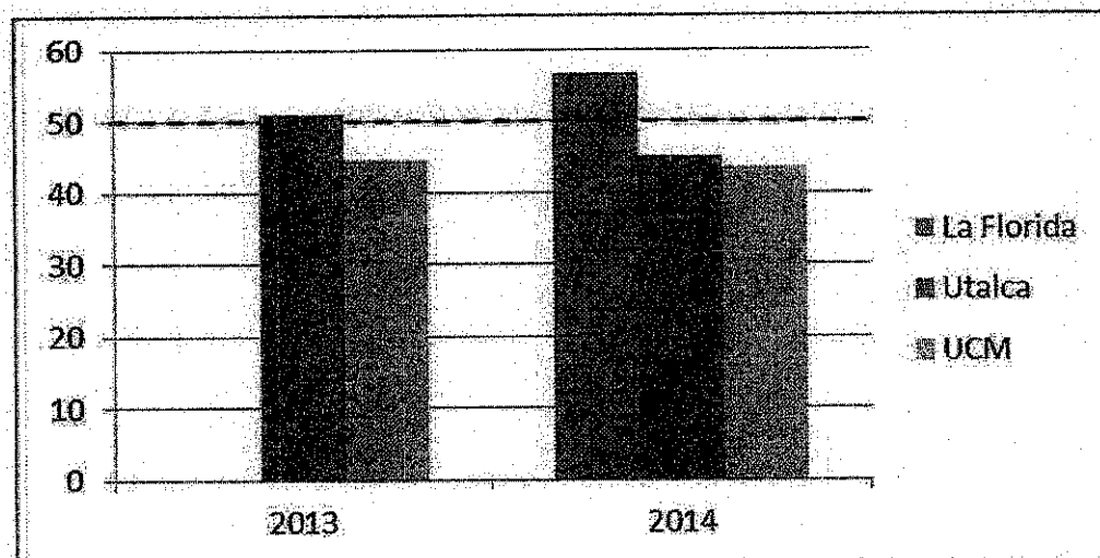
Figura 7. Concentraciones anuales MP10
