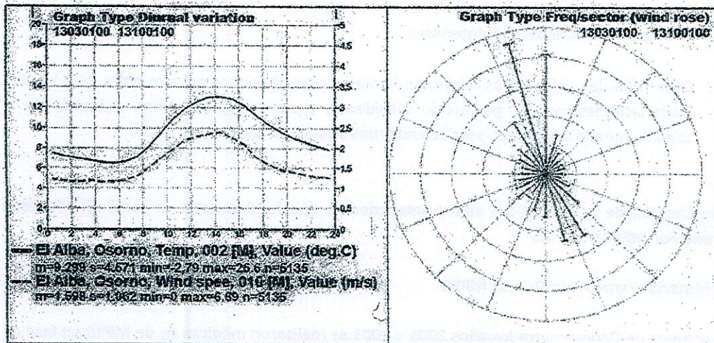
Figura 1. Variación diaria en temperatura y velocidad del viento (izquierda) y rosa de los vientos (derecha) de Estación El Alba. Resultado para el periodo 01-03-2013 al 30-09-2013.
