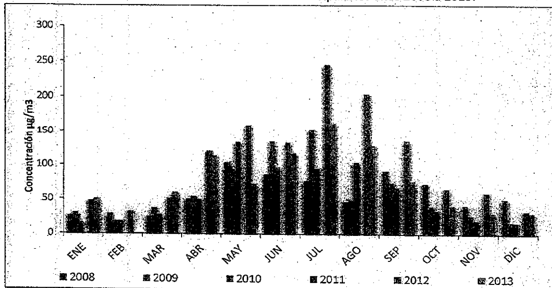
Figura 2: Distribución anual de la concentración de MP10 para los años 2008 a 2013.
