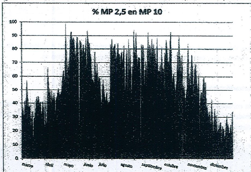
Figura 6. Distribución anual del % de concentración de MP2,5 en MP10 (año 2013)
