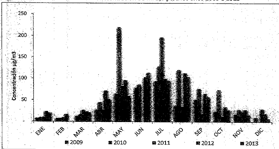
Figura 4: Distribución anual de la concentración de MP 2,5 para los años 2009 a 2013
