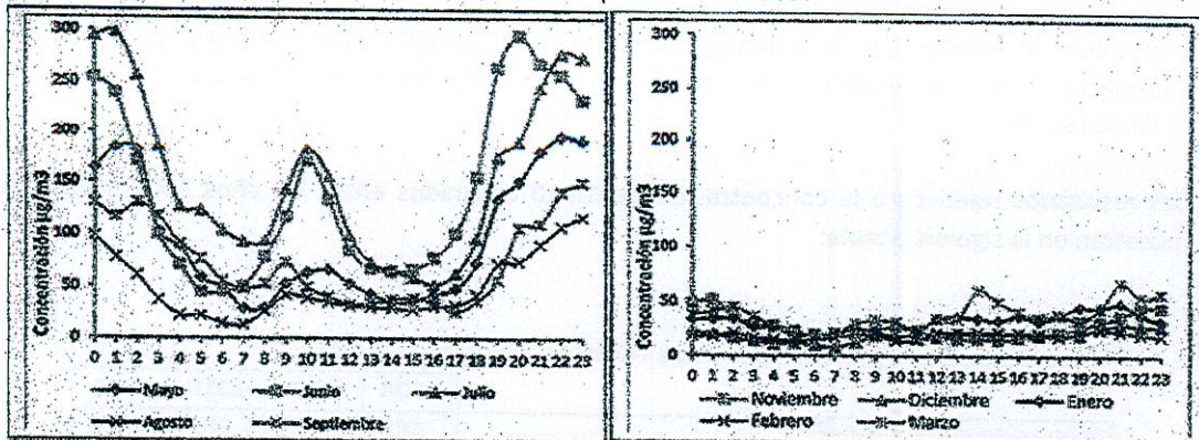
Figura 3: Ciclo de concentración diaria de MP10 para el año 2009.
