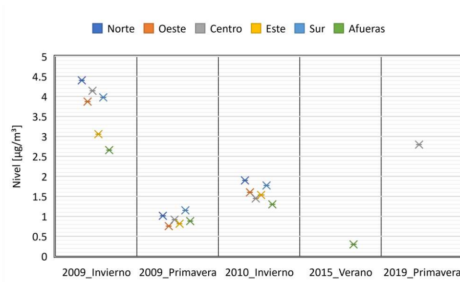
Figura 22: Gráfica Nivel de benceno en función de las Estaciones del año, identificando zona Norte, Oeste, Centro, Este, Sur y Afuera de la Provincia de Santiago.
