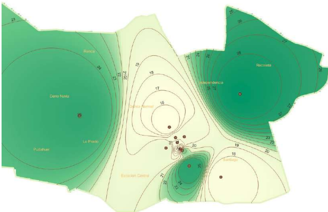
Figura 3.2: Tolueno
