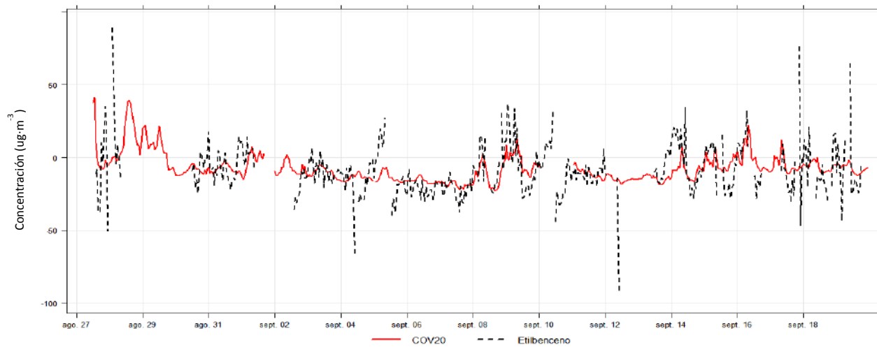
Figura 3.21. Serie temporal de salida de modelo para sensor COV_20 en unidades de \mu\text{g}\cdot\text{m}^{-3} , junto con concentración dada por el instrumento DOAS para el gas etilbenceno.
