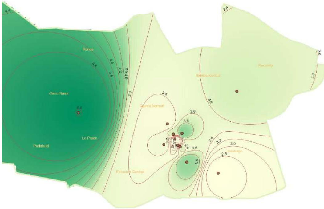
Figura 3.1: Benceno
