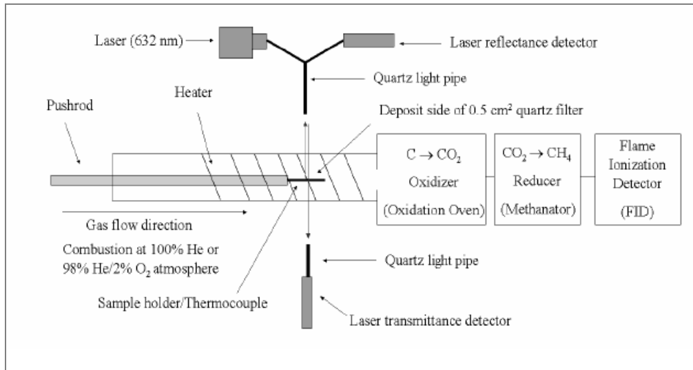
Figura 95: Horno de combustión, carga de la muestra, horno de oxidación, reductor cámara de ionización y sistema óptico.
