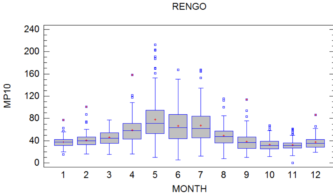
Figura 18: Perfil promedio anual de concentraciones de MP 10 (µg/m 3 ) en Rengo. Se incorporan datos entre el 2007 y 2011.
