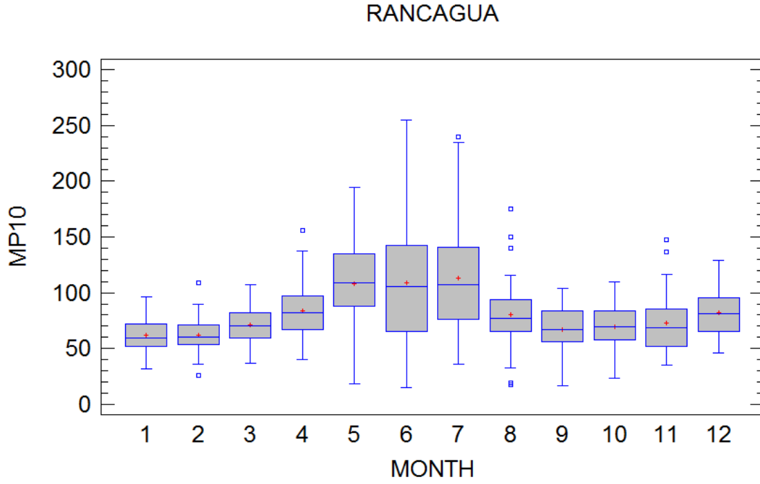
Figura 15: Perfil promedio mensual de MP 10 (µg/m 3 ) en la estación de Rancagua Histórica (promedios diarios). Datos incorporan mediciones simultáneas entre 2009-2011.
