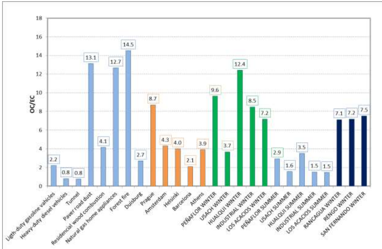
Figura 58: Relación Carbono Orgánico- Carbono Elemental (OC/EC) para distintas ciudades y fuentes emisoras.
