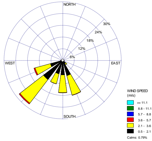
Figura 29: Rosa de vientos, estación San Fernando, período Nov-Feb (2009-2012)
