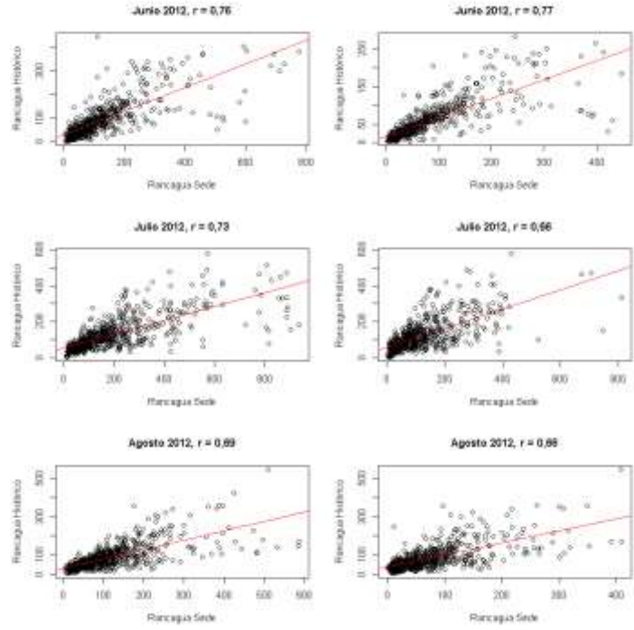
Figura 100: Ajustes lineales de MP_{10} (izquierda) y MP_{2.5} (derecha) y coeficiente de correlación r entre Rancagua Sede y Rancagua histórico (concentraciones en \mu g/m^3 ) durante el período Junio-Agosto 2012.
