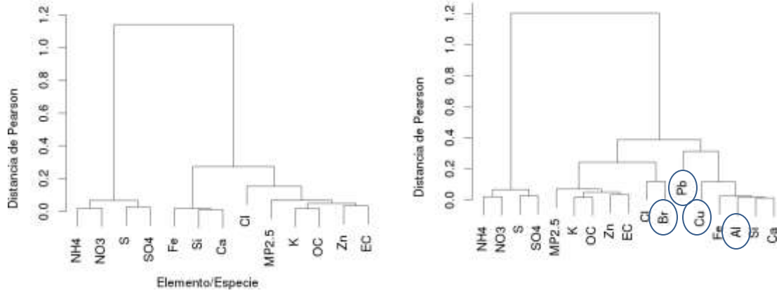
Figura 60. Conglomerados series de concentraciones de elementos, MP 2.5 iones OC y EC en Rancagua.
