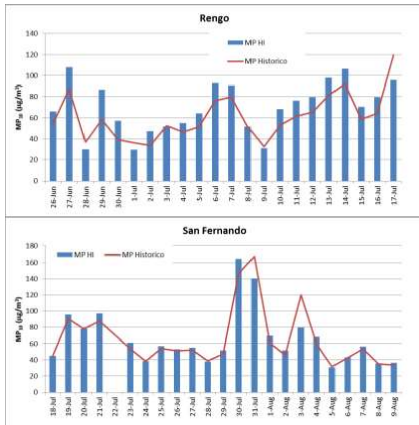
Figura 55: Series de tiempo de concentración de MP_{10} para la estación de Rengo (arriba) y San Fernando (abajo). Líneas indican monitoreo continuo oficial, barras indican monitoreo con Impactadores de Harvard (HI). Los datos son concentración de 24 hrs promedio
