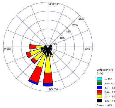
Figura 27: Rosa de vientos, estación Rengo, período Nov-Feb (2009-2012)
