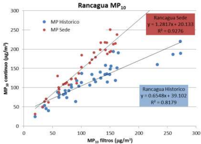
Figura 4: Correlación para MP 10 entre instrumentos continuos y discretos, en Rancagua.
