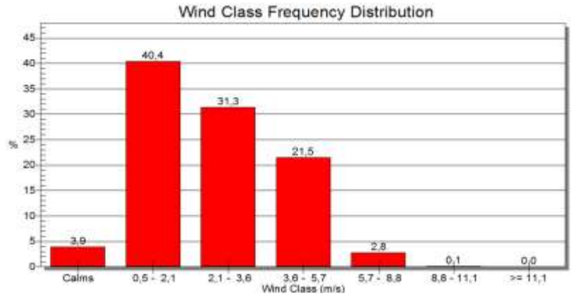
Figura 46: Vientos estación Sewell
