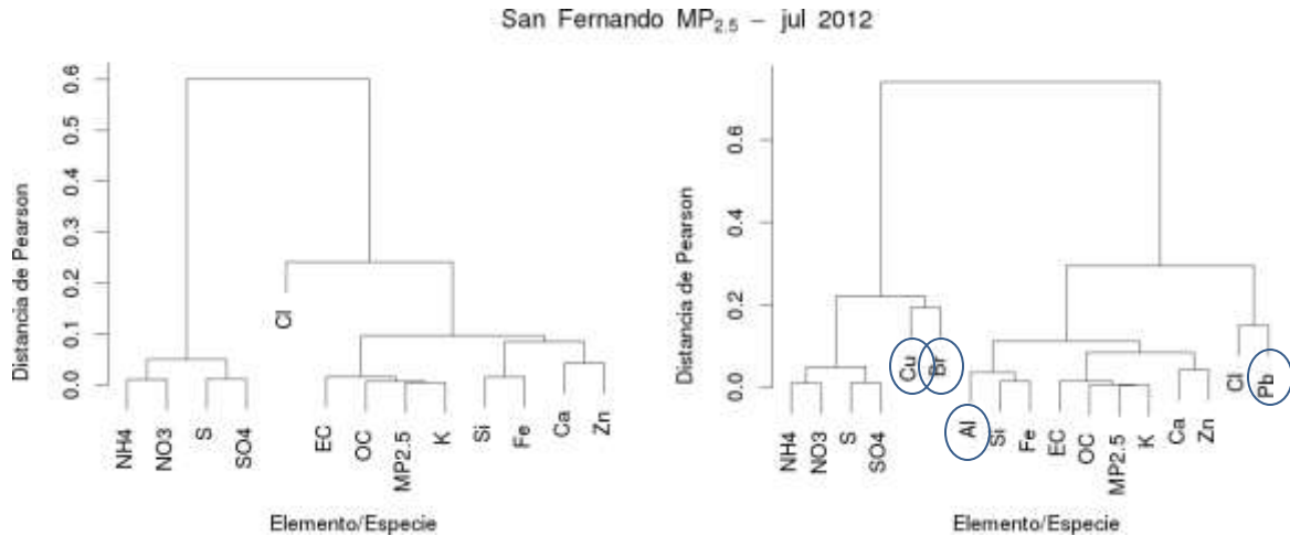
Figura 62: Conglomerados series de concentraciones de elementos, MP_{2.5} iones OC y EC en San Fernando.
