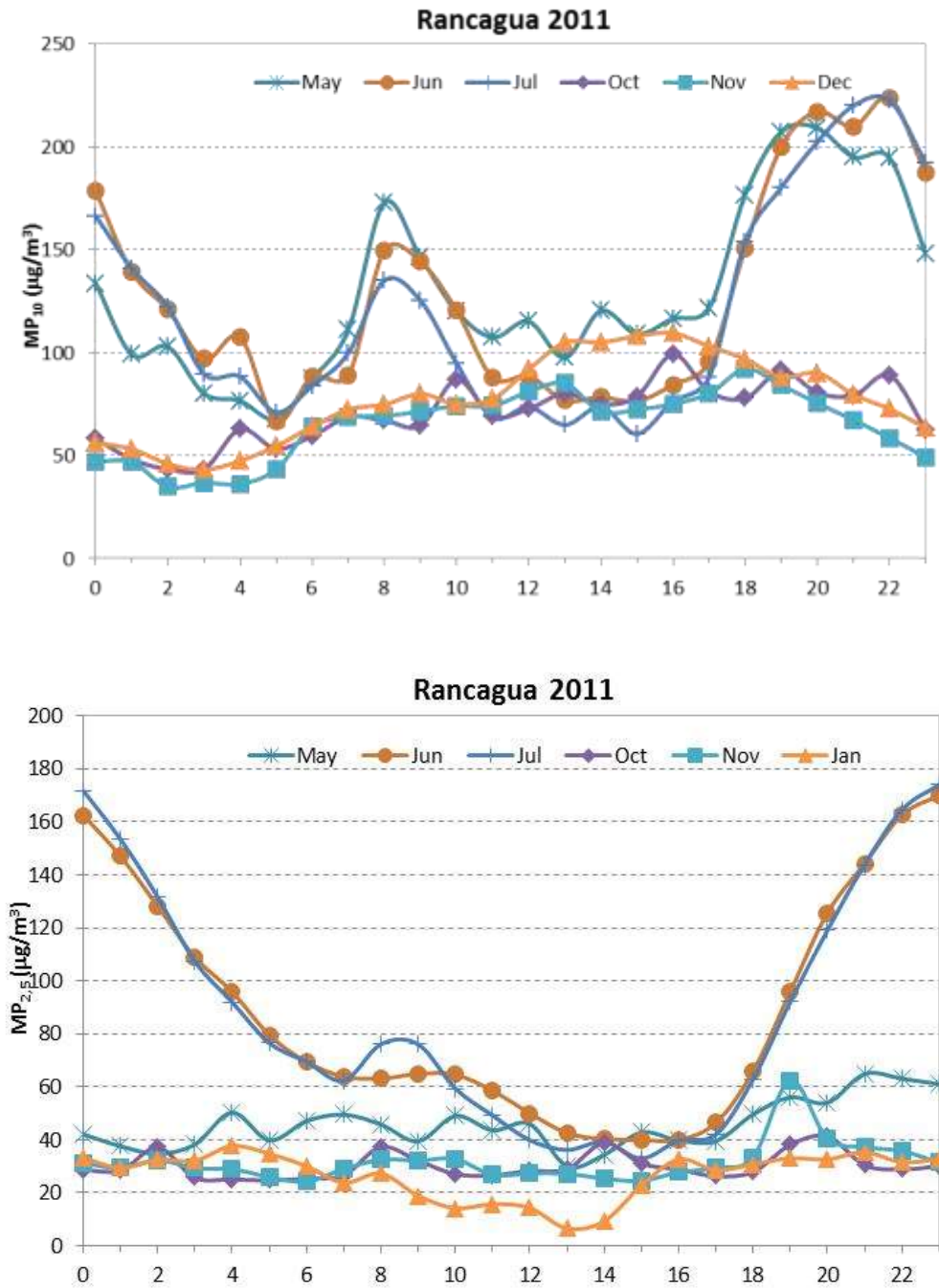
Figura 16: Perfiles promedios horarios de concentración de MP 10 y MP 2,5 para algunos meses del año 2011.
