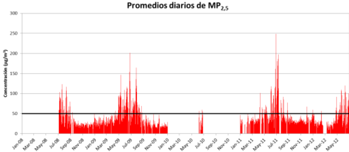
Figura 13: Concentraciones promedios diarias para MP_{2,5} estación de Rancagua histórica.
