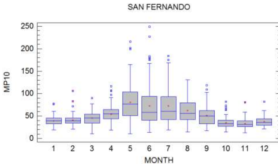
Figura 21: Perfil promedio anual de concentraciones de MP_{10} ( \mu\text{g}/\text{m}^3 ) en San Fernando. Mediciones entre los años 2007-2011.
