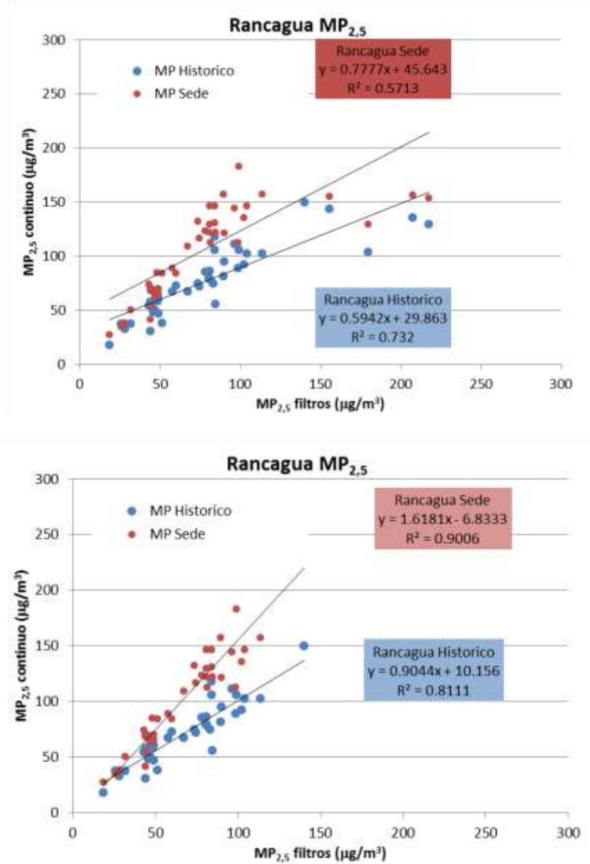
Figura 5: Correlación para MP 2,5 entre instrumentos continuos y discretos, en Rancagua. Arriba se muestra la serie completa de datos, abajo se han eliminado valores de concentración altas medidas por HI.
