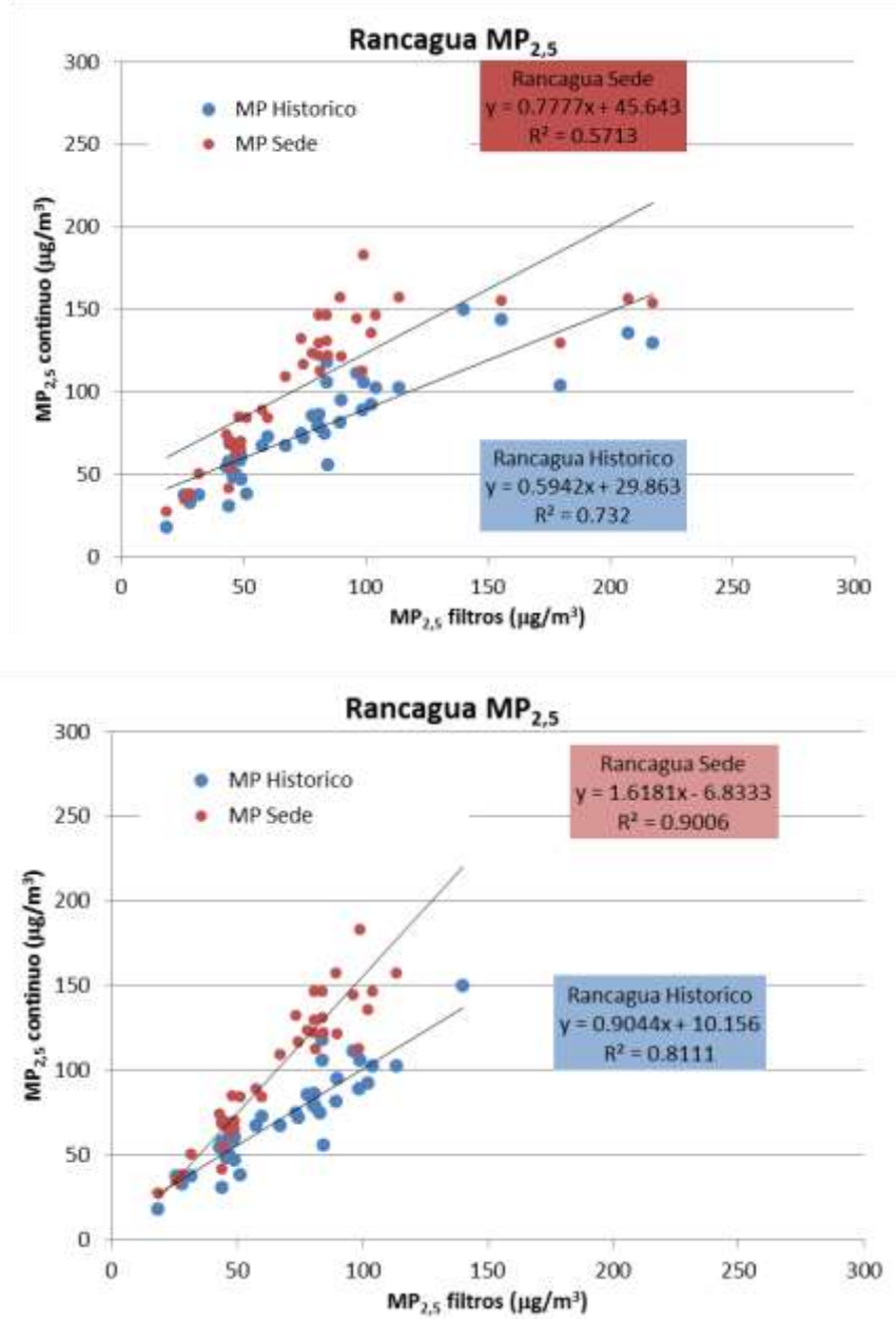
Figura 54: Correlación para MP 2,5 entre instrumentos continuos y discretos, en Rancagua. Arriba se muestra la serie completa de datos, abajo se han eliminado valores de concentración altas medidas por HI.
