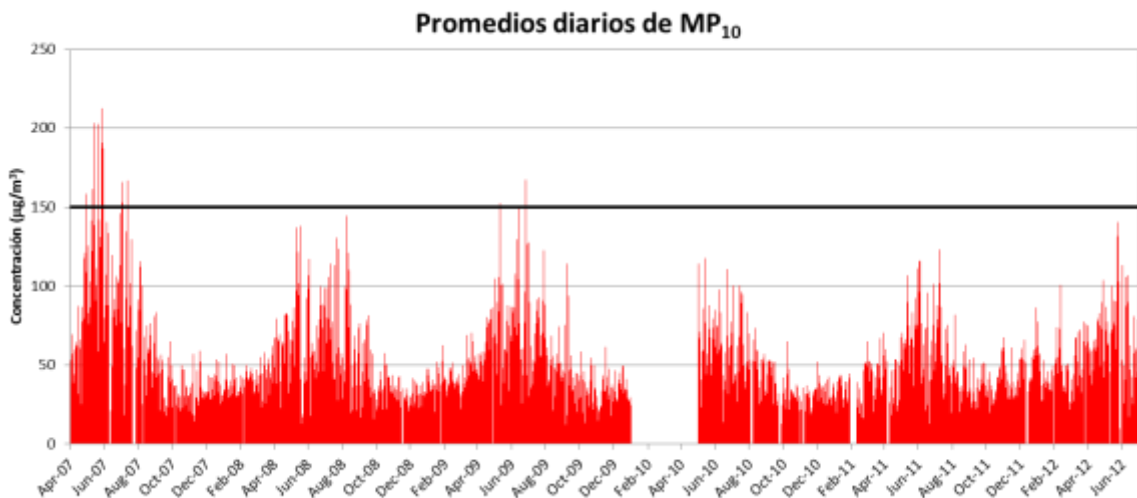
Figura 17: Promedios diarios de concentración de MP_{10} .
