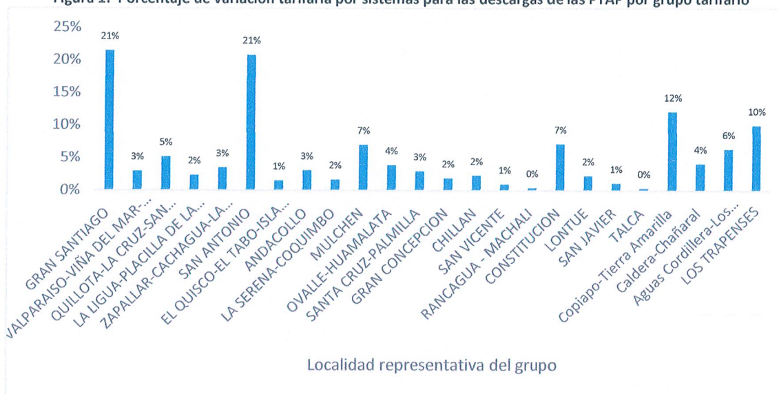
Figura 1: Porcentaje de variación tarifaria por sistemas para las descargas de las PTAP por grupo tarifario
