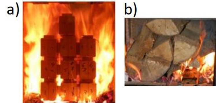
Figura 1: Ejemplo de los métodos de testeo, a) Crib Wood; b) Cord Wood.
