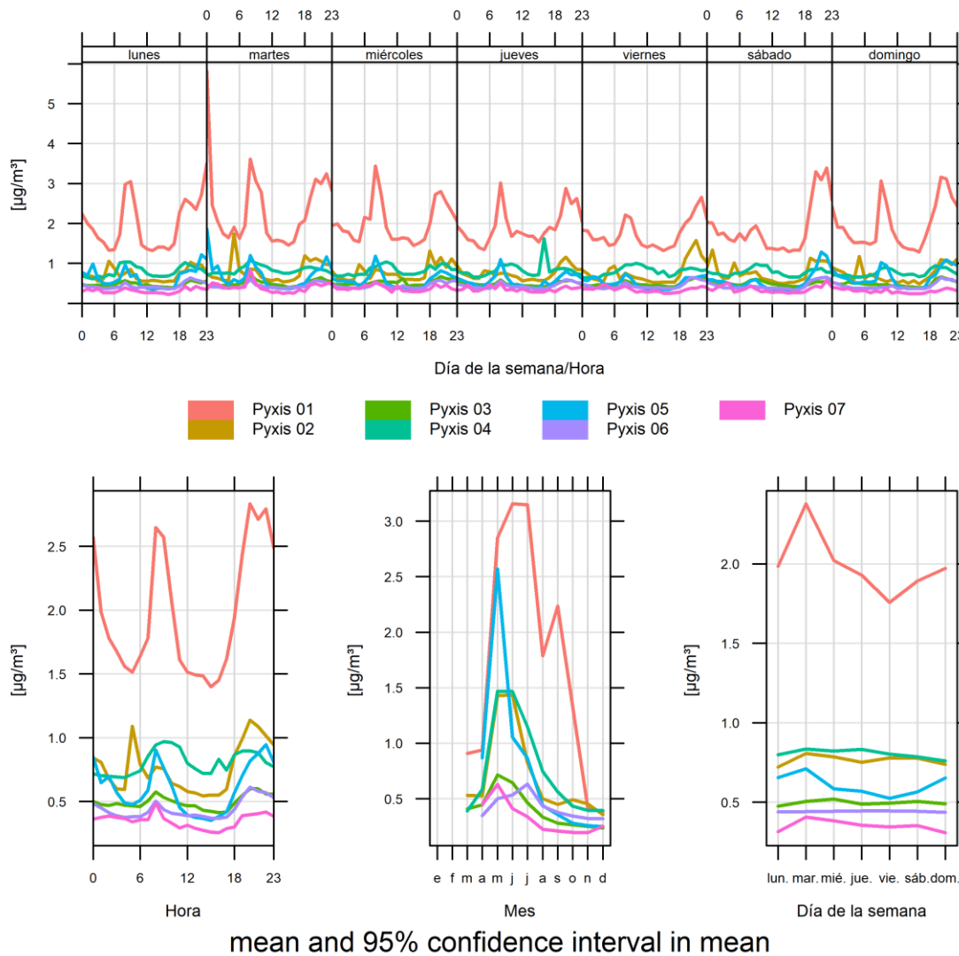
Figura 12: Variabilidad temporal de concentraciones de benceno para equipos PyxisGC - 2023
