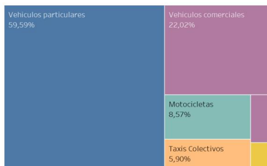
Figura 5-36 Emisiones CO de fuentes móviles para Región Metropolitana de Santiago Año 2019
