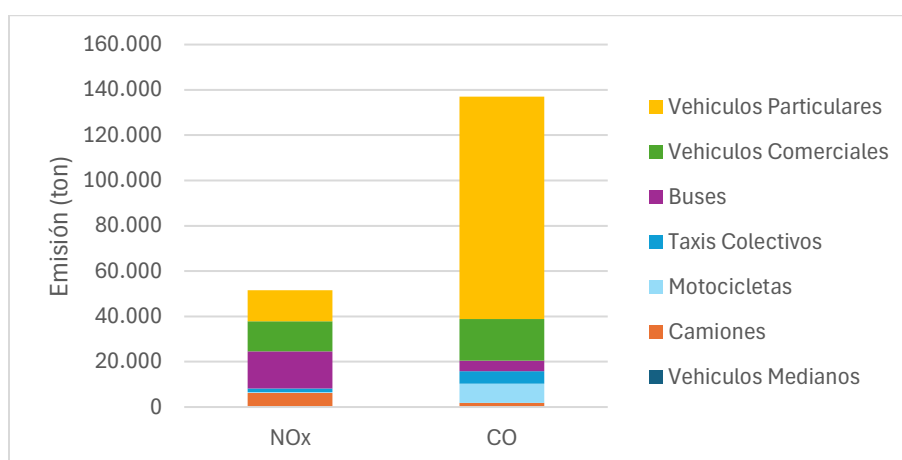
Figura 5-32 Emisiones de NO x y CO de fuentes móviles por tipo de vehículos año 2019 (ton)
