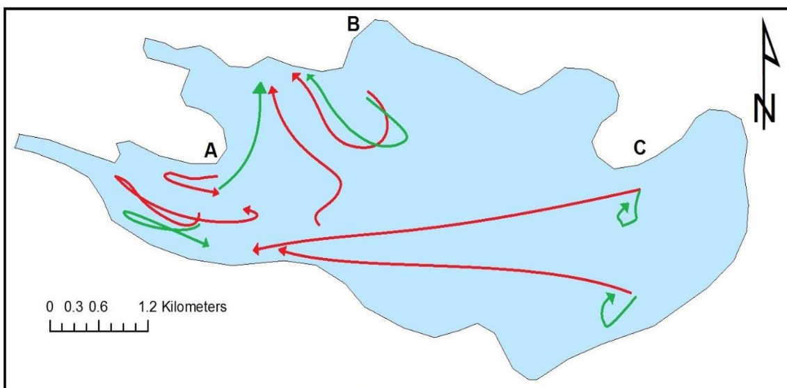
Figura 49. Mediciones de correntometr3a en el tramo A, B y C del lago Huillenco. Color verde= correntometr3a de profundidad, color rojo= correntometr3a de superficie.
