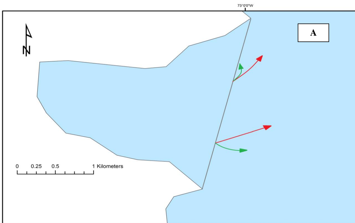
Figura 22. Lago Llanquihue: Dirección de las corrientes medidas mediante correntometría lagrangeana en cada bahía a 1 m (rojo) y 15 m (verde) de profundidad. A= Phillipi, B= Maitén, C= Frutillar, D= Rincones, E= Puerto Octay, F= Puerto Fonck, G= Bahía Ensenada, H= Bahía Volcán.
