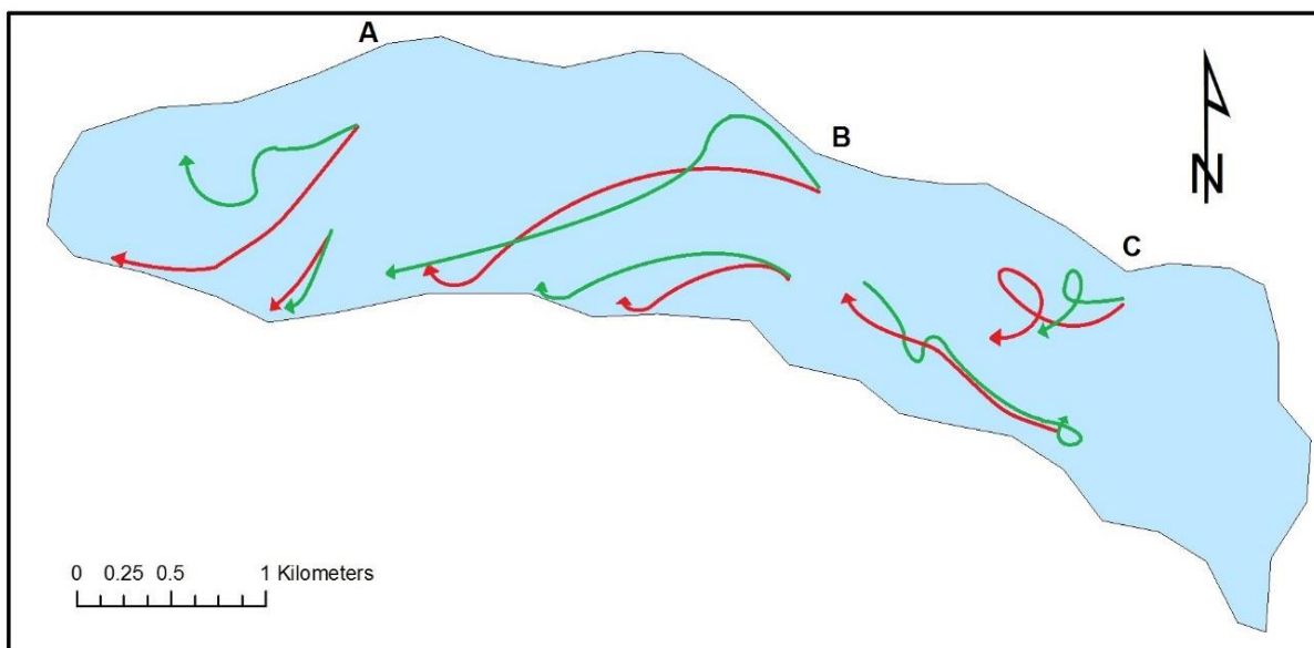
Figura 40. Mediciones de correntometría en el tramo A, B y C del lago Natri. Color verde= correntometría de superficie, color rojo= correntometría de profundidad.
