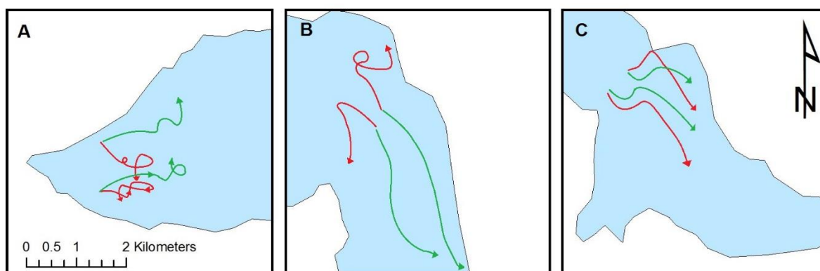
Figura 31. Mediciones de correntometría en el tramo A, B y C del lago Chapo. Color verde= correntometría de superficie, color rojo= correntometría de profundidad.
