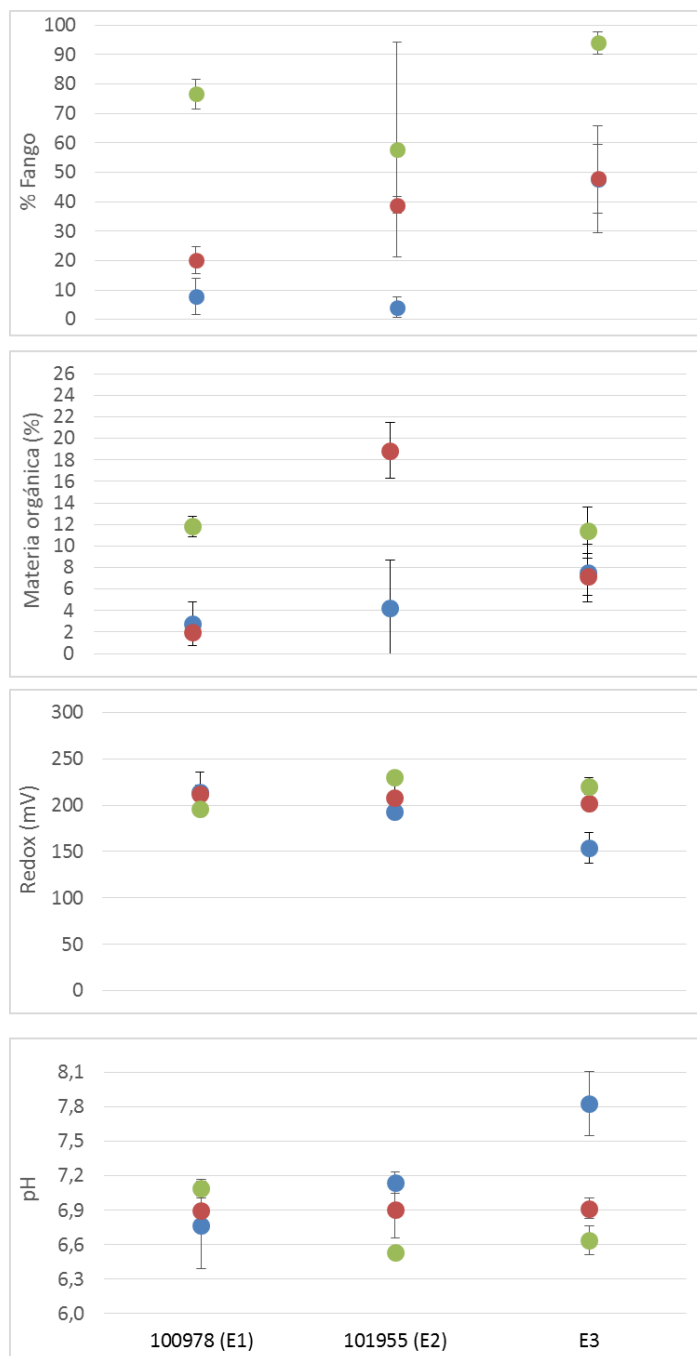
Figura 75. Lago Ranco: valores promedio y desviaci3n est3ndar de fango (%), materia org3nica (%), redox (mV) y pH en sedimentos para las diferentes estaciones de muestreo. E1 y E2 corresponden a las concesiones 100978 y 101955, respectivamente.
