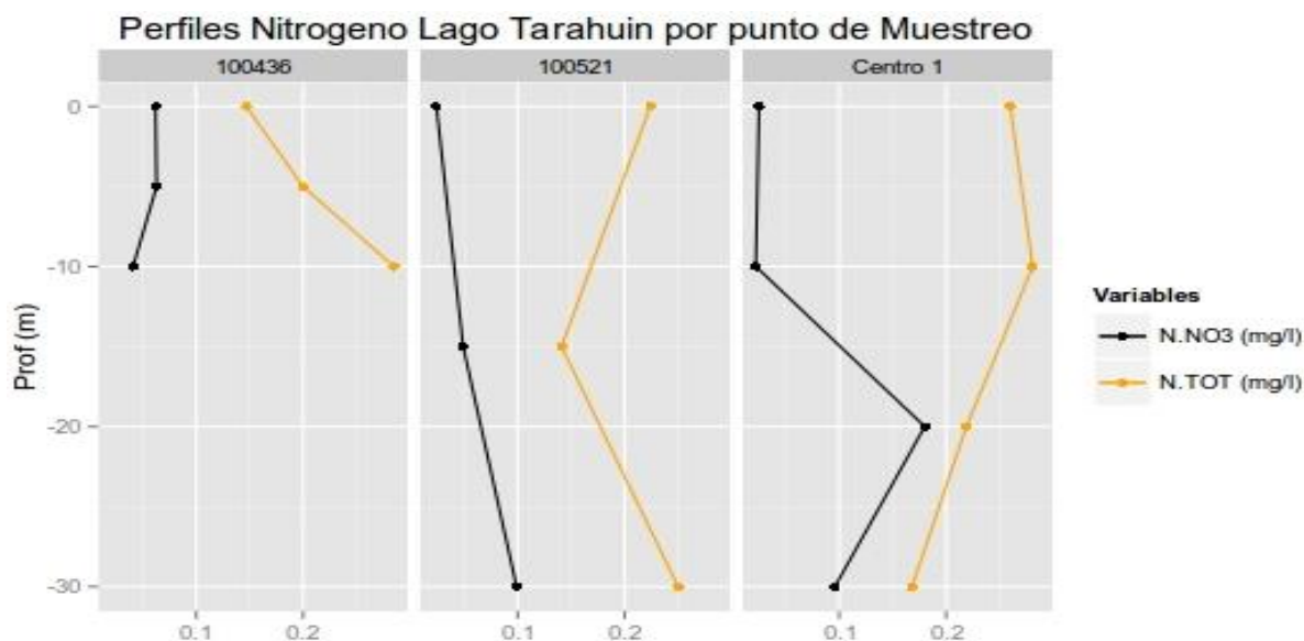
Figura 52. Perfiles de compuestos nitrogenados (N-NO 3 en mg/L y NT en mg/L) en los centros analizados en el lago Tarahuín.
