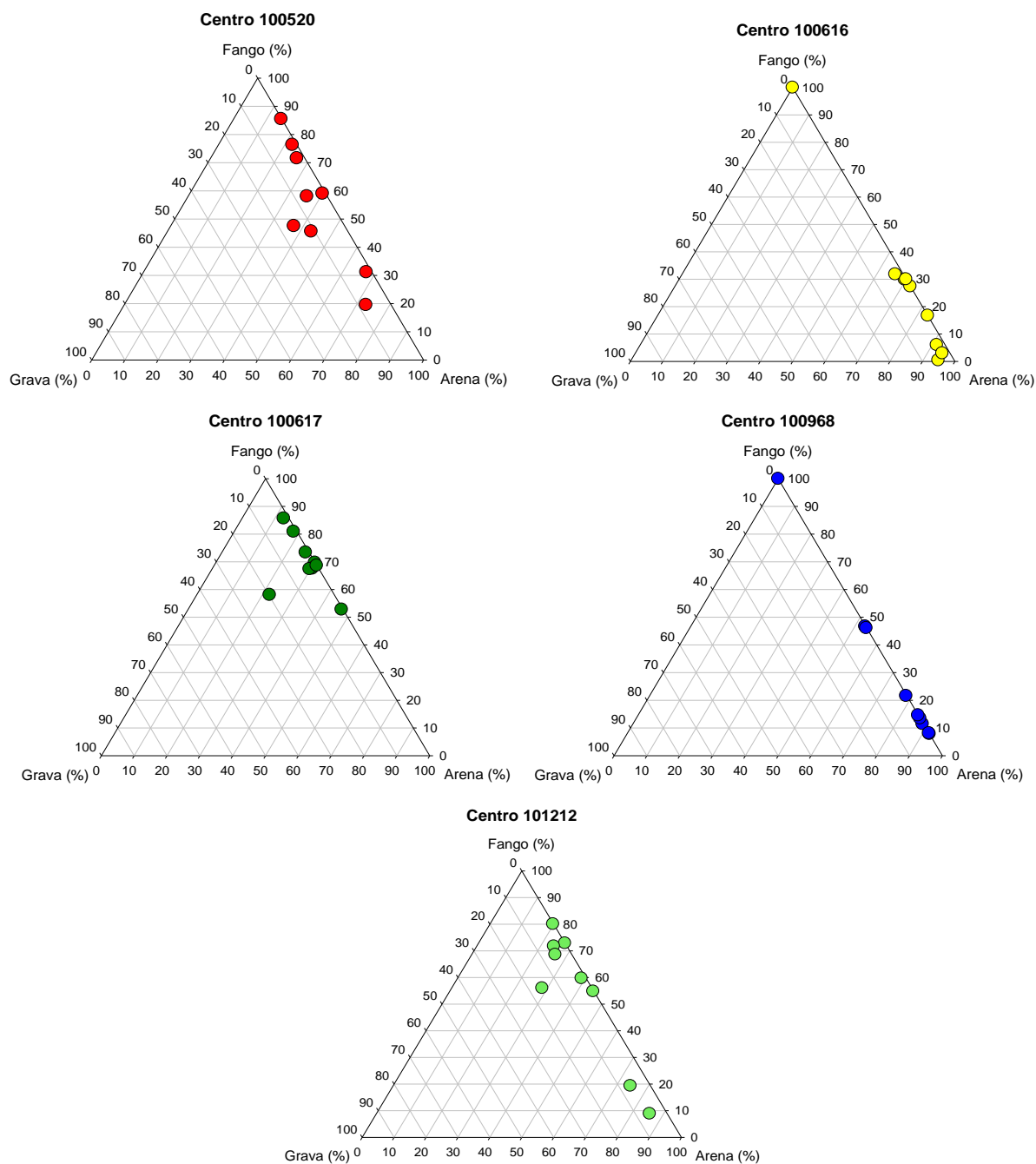
Figura 46. Lago Huillenco: Fracciones texturales (% fango, % arena y % grava) representadas en un gr3fico de tri3ngulo para cada centro.
