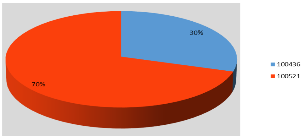
Figura 121. Producci3n hist3rica (%) por centro de cultivo en el lago Tarahu3n.
