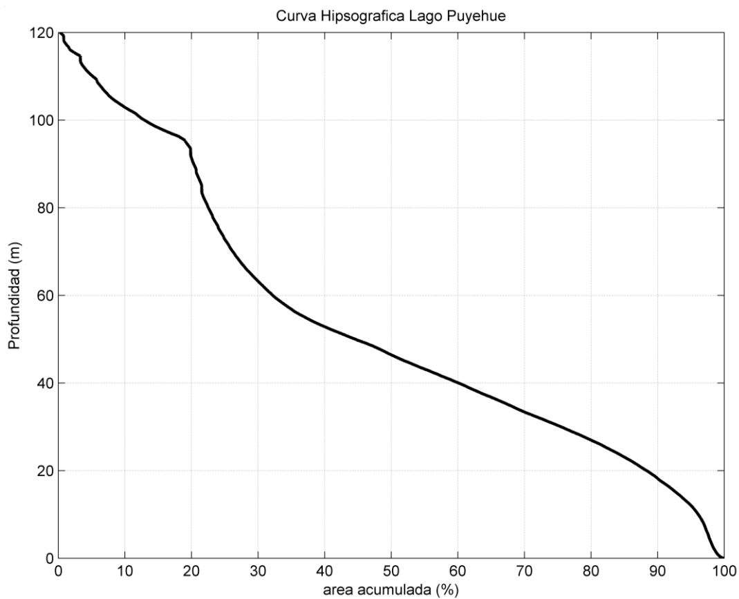
Figura 3. Curva hipsográfica lago Puyehue.
