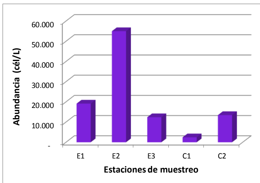
Figura 90. Abundancia fitoplanct3nica (c3l/L) en las estaciones de muestreo del lago Puyehue, durante la primavera de 2014.
