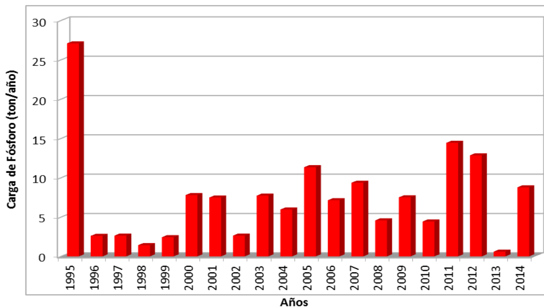
Figura 112. Aporte de PT (ton/año) desde centros de cultivo en el lago Natri.
