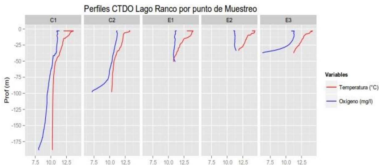
Figura 68. Perfiles físico-químicos (oxígeno en mg/L, y temperatura en °C) de la columna de agua en los centros analizados en el lago Ranco (E1 corresponde a la concesión 100978, y E2 a 101955).
