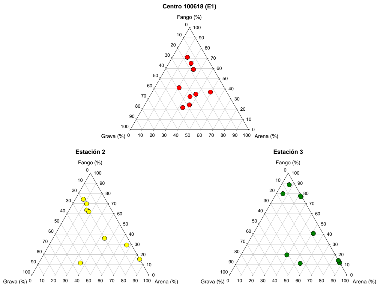
Figura 64. Lago Cucao: Fracciones texturales (% fango, % arena y % grava) representadas en un gráfico de triángulo para cada centro.
