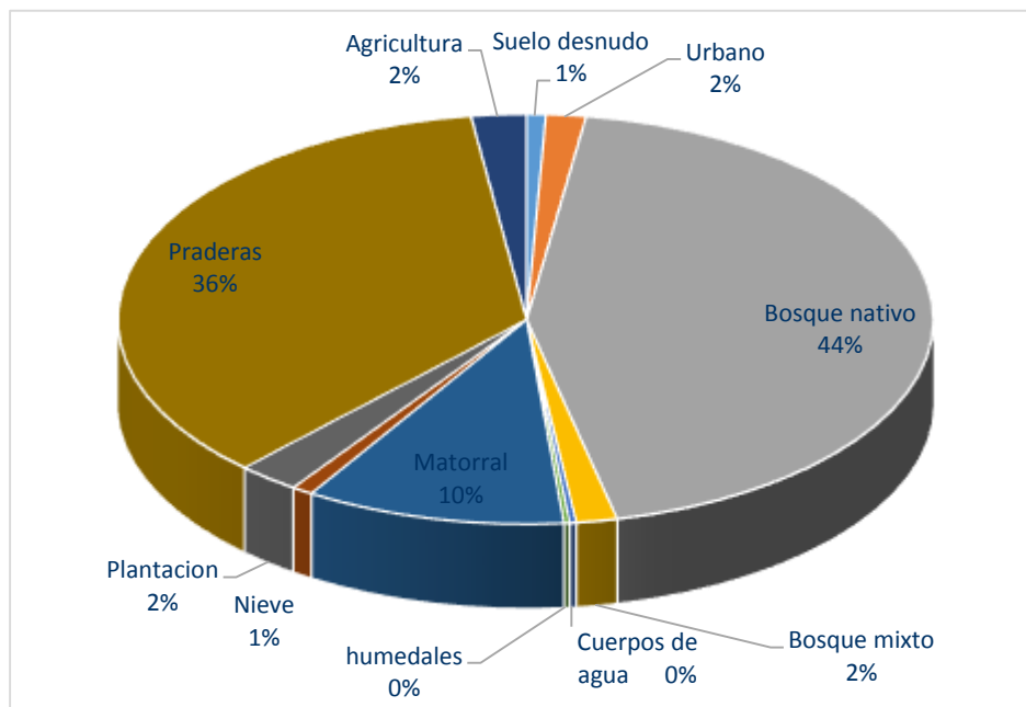
Figura 97. Uso de suelo (%) en la cuenca del lago Llanquihue.
