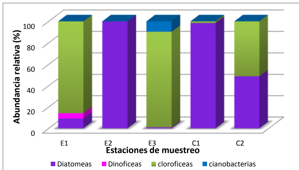
Figura 89. Abundancia relativa (%) en las estaciones de muestreo del lago Puyehue, durante la primavera de 2014.
