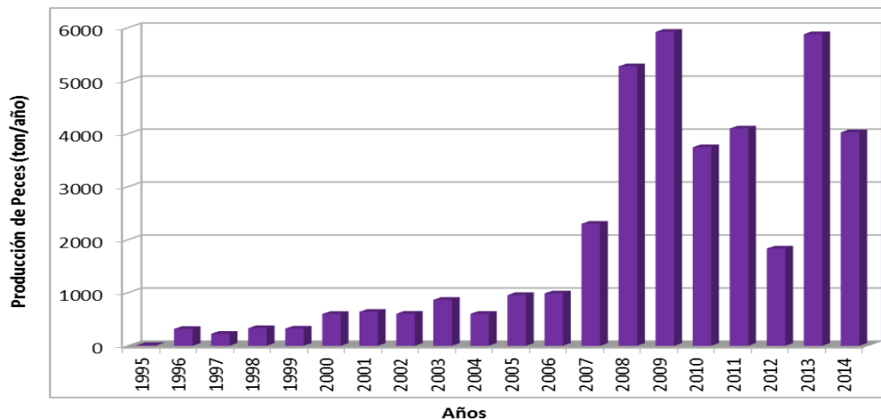
Figura 137. Producci3n hist3rica de peces (ton/a3o) en el lago Puyehue.
