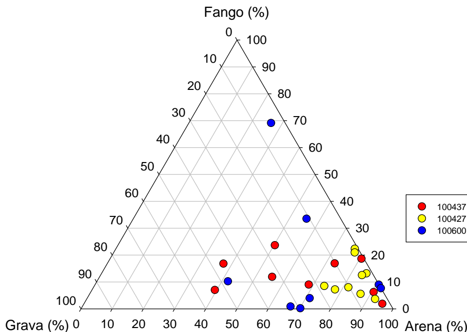
Figura 38. Lago Natri: Gráfico de triángulo para clasificación de textura (% fango, % arena y % grava).
