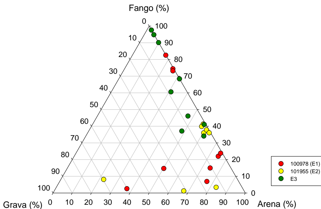
Figura 74. Lago Ranco: Gráfico de triángulo para clasificación de textura (% fango, % arena y % grava).
