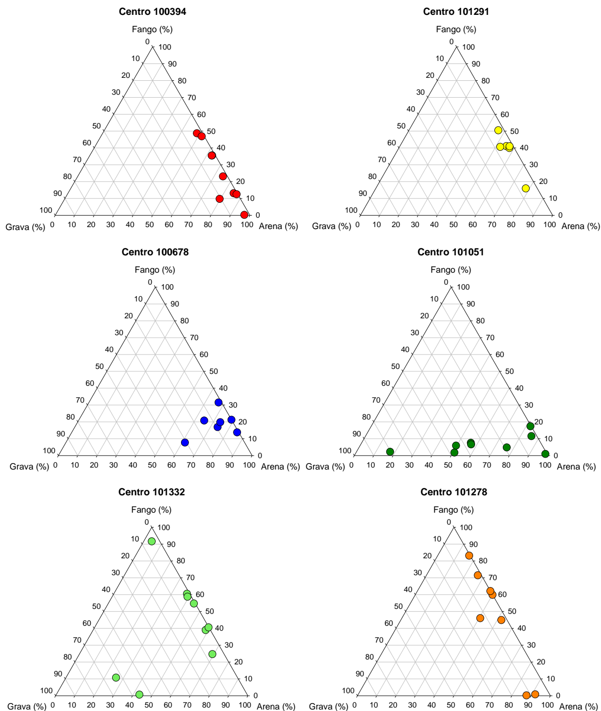
Figura 28. Lago Chapo: Fracciones texturales (% fango, % arena y % grava) representadas en un gr3fico de tri3ngulo para cada centro.
