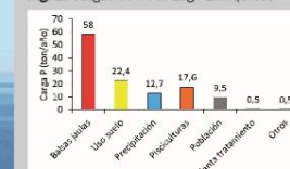
Fig. 2: Cargas de PT al Lago Llanquihue
