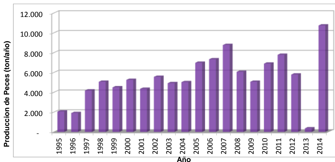
Figura 99. Producción histórica de peces (ton/año) en el lago Llanquihue.
