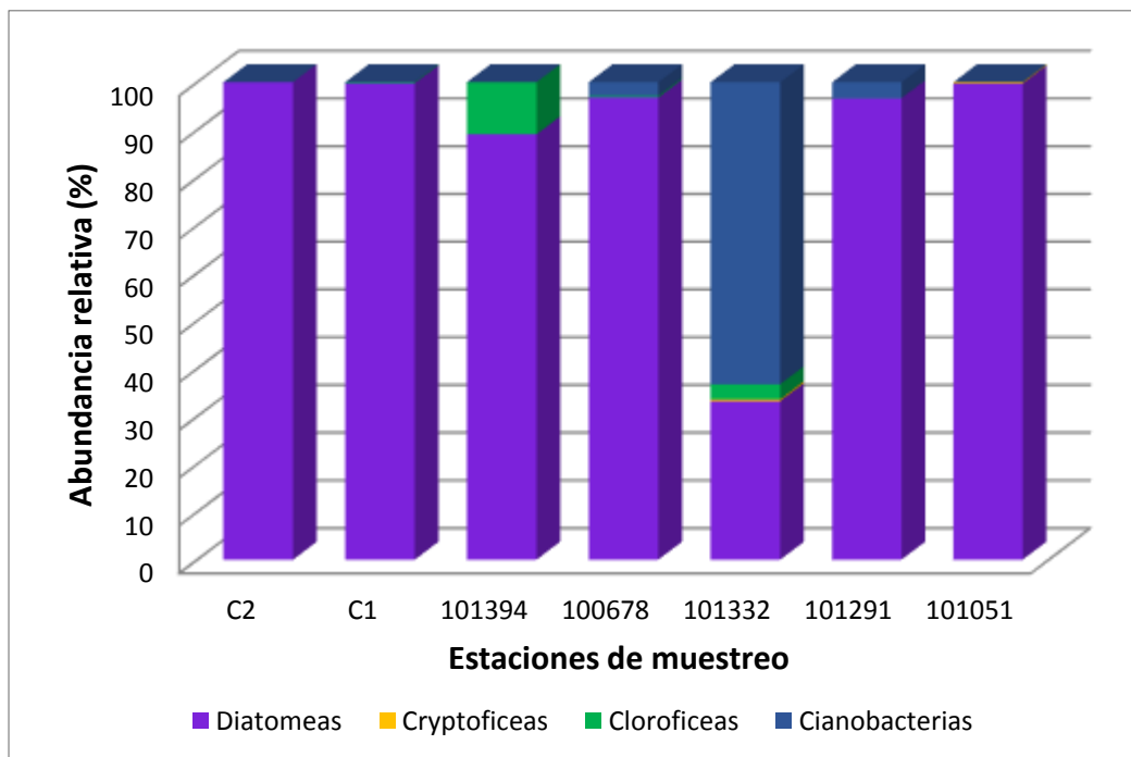
Figura 27. Abundancia relativa (%) en las estaciones de muestreo del lago Chapo, durante el otoño de 2014.
