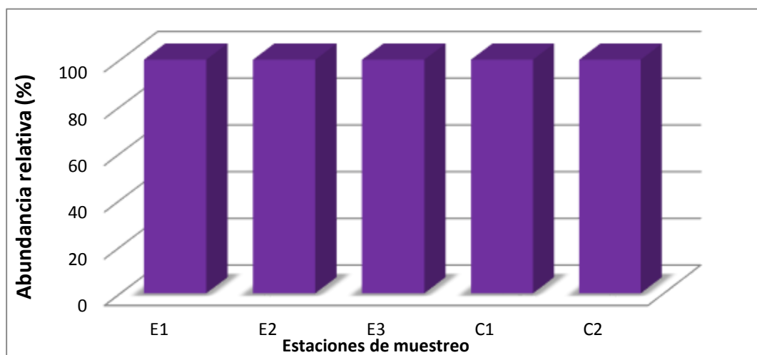
Figura 62. Abundancia relativa (%) en las estaciones de muestreo del lago Cucao, durante el invierno de 2014.
