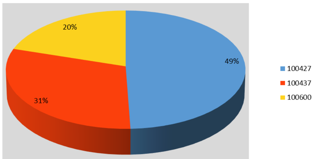
Figura 111. Producción histórica (%) por centro de cultivo en el lago Natri.
