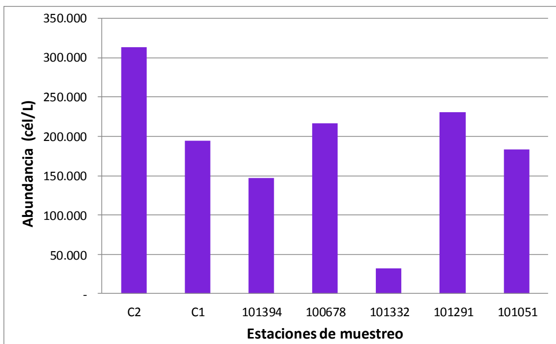
Figura 26. Abundancia fitoplanct3nica (cél/L) en las estaciones de muestreo del lago Chapo, durante el otoño-invierno de 2014.
