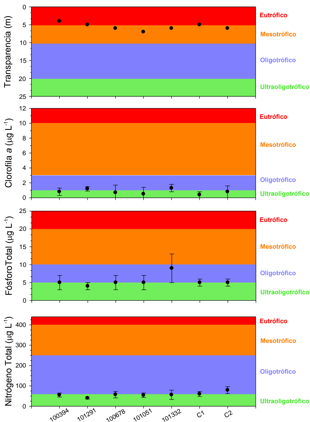
Figura 104. Indicadores tróficos: Transparencia (m), clorofila a ( \mu\text{g L}^{-1} ), fósforo total ( \mu\text{g L}^{-1} ) y nitrógeno total ( \mu\text{g L}^{-1} ) en lago Chapo.
