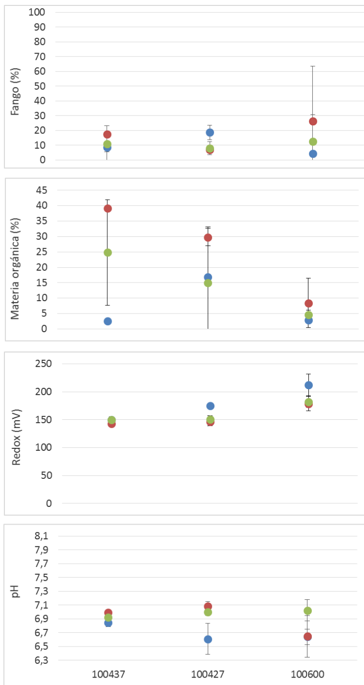
Figura 39. Lago Natri: valores promedio y desviaci3n estandar de fango (%), materia orgánica (%), redox (mV) y pH en sedimentos para las diferentes estaciones de muestreo.
