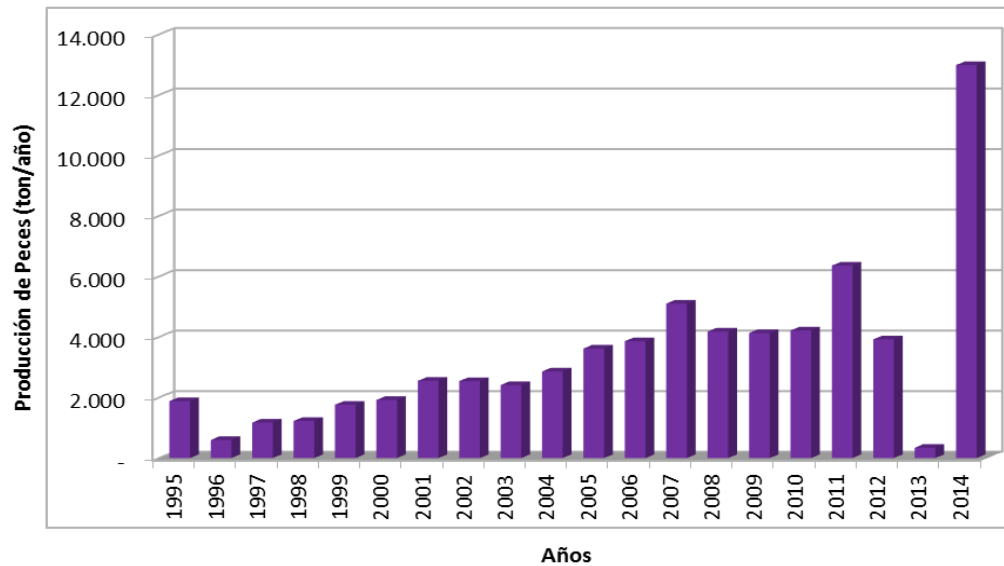
Figura 129. Producci3n hist3rica de peces (ton/a3o) en el lago Rupanco.
