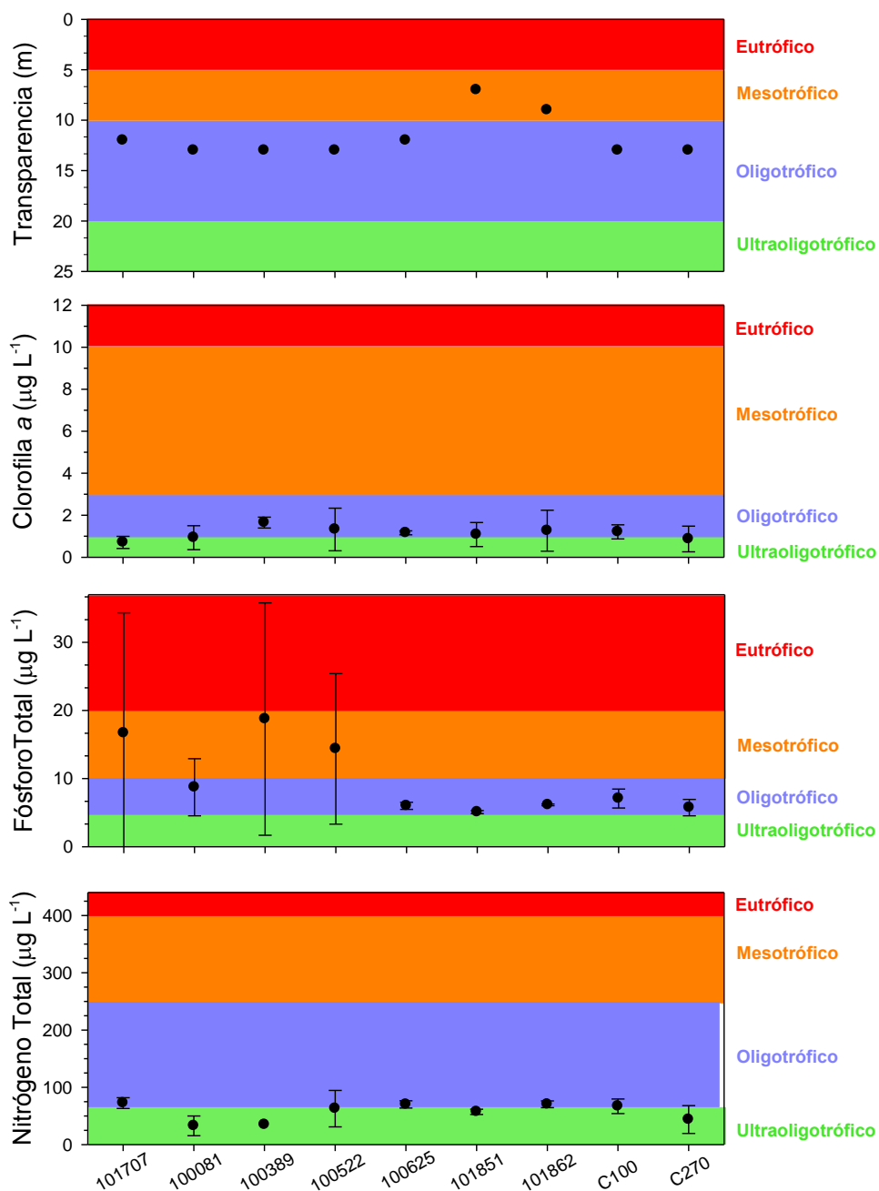
Figura 128. Indicadores tróficos: Transparencia (m), clorofila a ( \mu\text{g L}^{-1} ), fósforo total ( \mu\text{g L}^{-1} ) y nitrógeno total ( \mu\text{g L}^{-1} ) en lago Rupanco.
