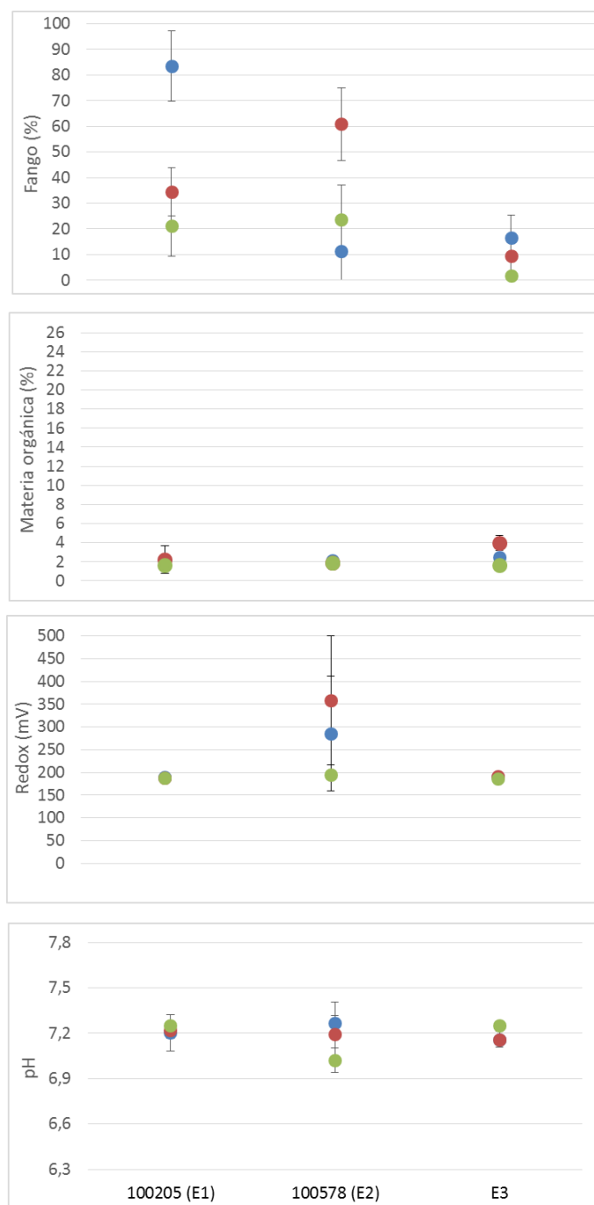
Figura 93. Lago Puyehue: valores promedio y desviaci3n est3ndar de fango (%), materia org3nica (%), redox (mV) y pH en sedimentos para las diferentes estaciones de muestreo. E1 y E2 corresponden a las concesiones 100205 y 100578, respectivamente.
