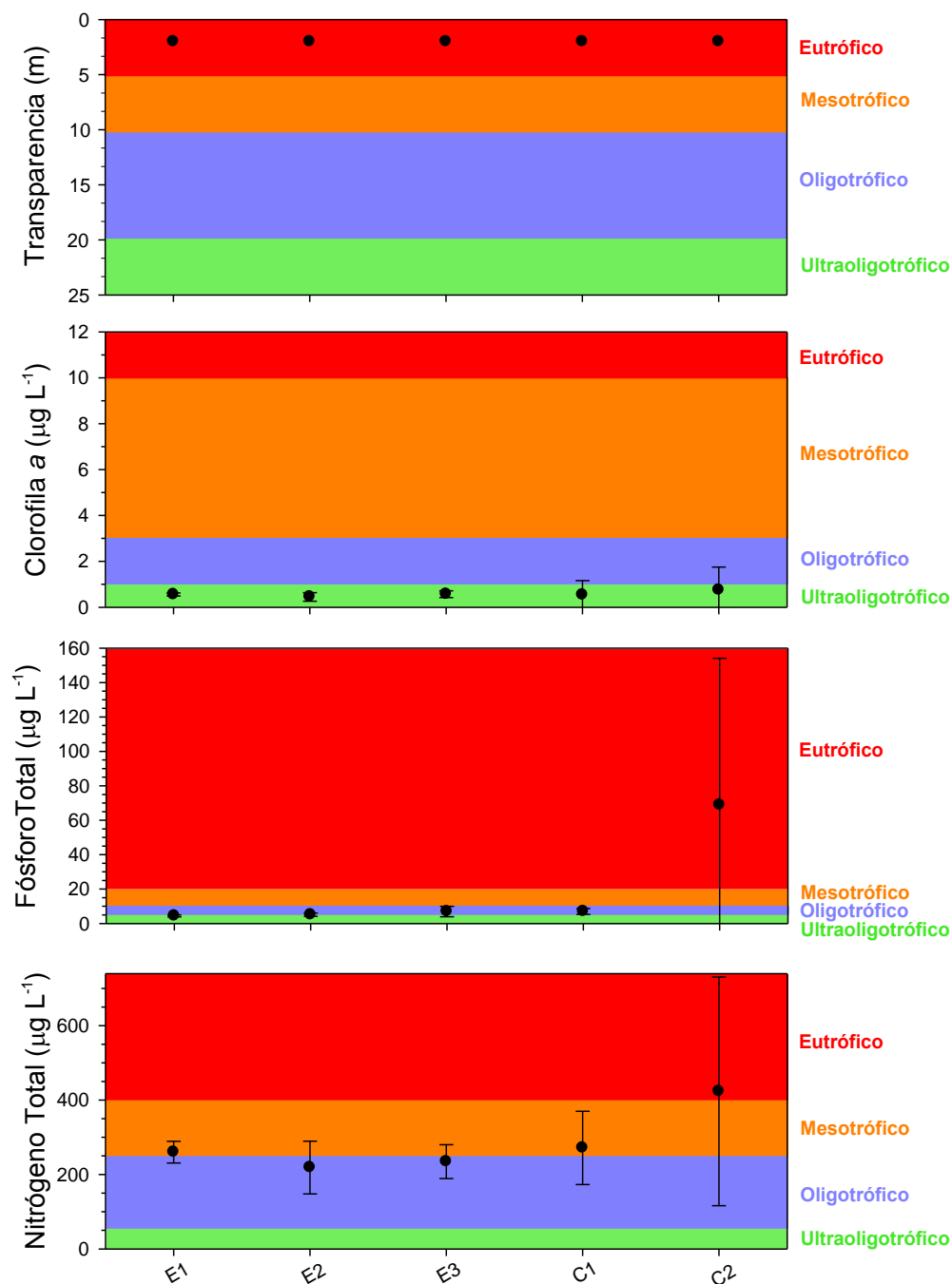
Figura 123. Indicadores tr3ficos: Transparencia (m), clorofila a ( \mu\text{g L}^{-1} ), f3sforo total ( \mu\text{g L}^{-1} ) y nitr3geno total ( \mu\text{g L}^{-1} ) en lago Cucao.
