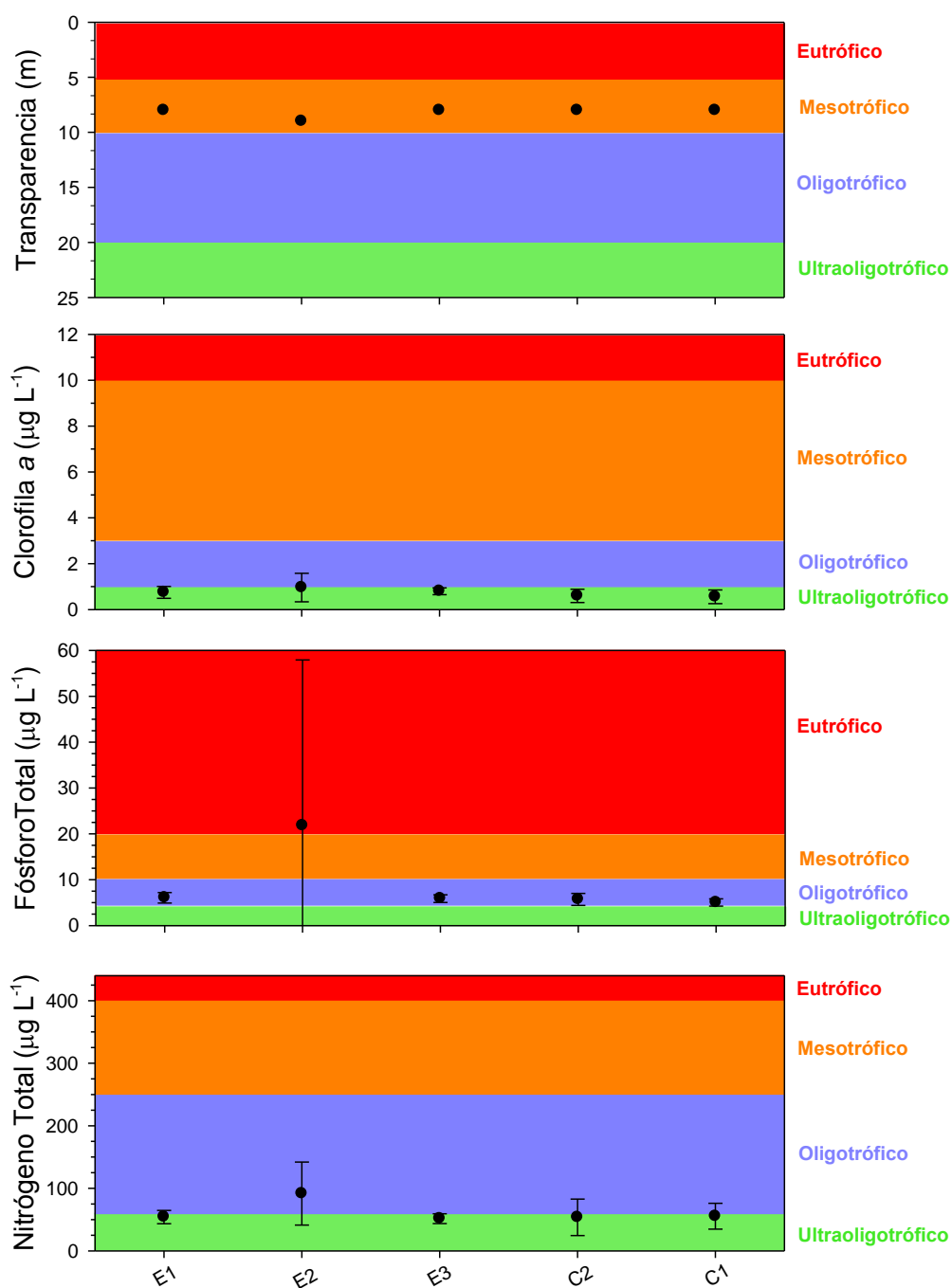
Figura 132. Indicadores tróficos: Transparencia (m), clorofila a ( \mu\text{g L}^{-1} ), fósforo total ( \mu\text{g L}^{-1} ) y nitrógeno total ( \mu\text{g L}^{-1} ) en lago Ranco.
