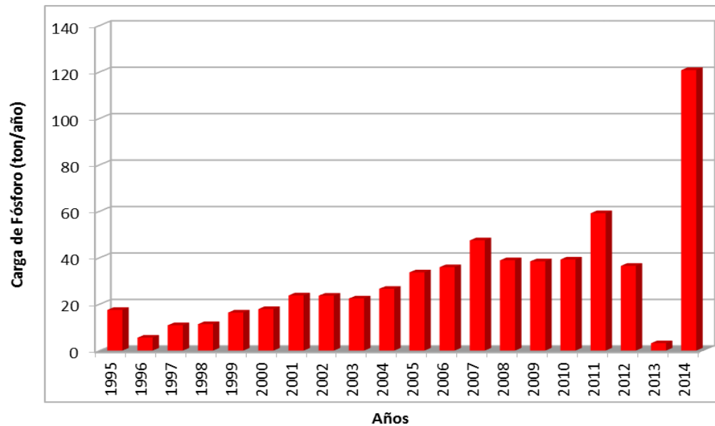
Figura 131. Aporte de PT (ton/a3o) desde centros de cultivo en el lago Rupancho.
