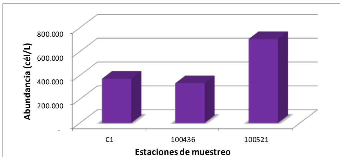
Figura 54. Abundancia fitoplanctónica (cél/L) en las estaciones de muestreo del lago Tarahuín, durante el invierno de 2014.
