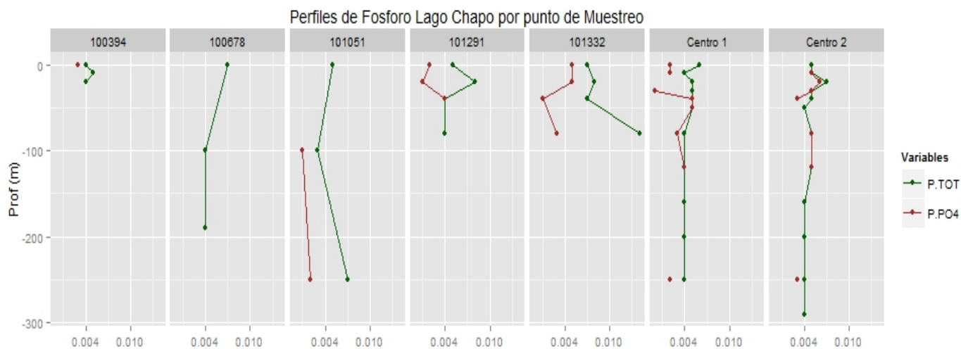
Figura 24. Perfiles de ortofosfato (P-PO 4 en mg/L) y fósforo total (PT en mg/L) de la columna de agua de los centros analizados en el lago Chapo (---P-PO 4 ; ---PT).
