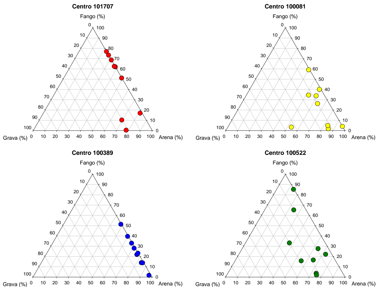
Figura 82. Lago Rupanco: Fracciones texturales (% fango, % arena y % grava) representadas en un gr3fico de tri3ngulo para cada centro.
