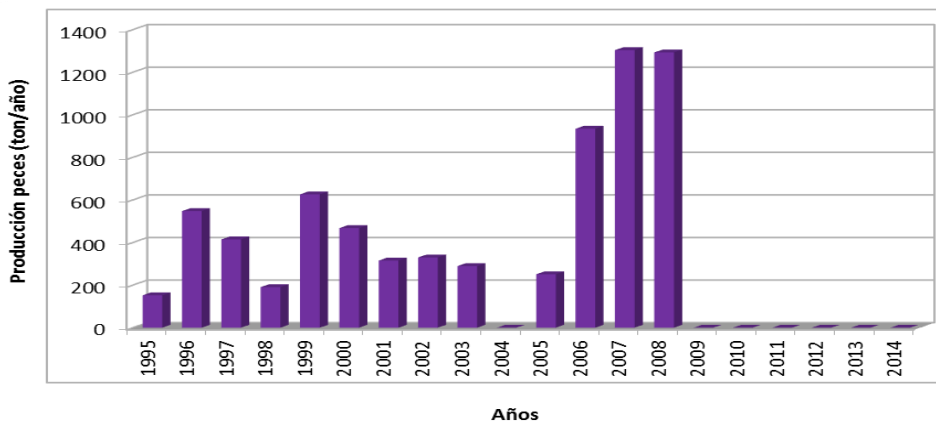
Figura 125. Producción histórica de peces (ton/año) en el lago Cucao.
