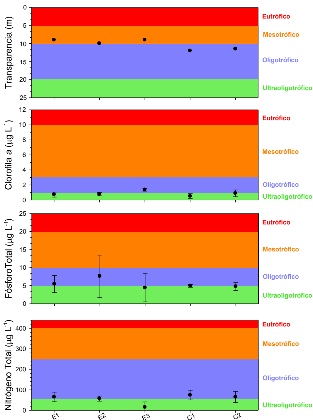
Figura 136. Indicadores tr3ficos: Transparencia (m), clorofila a ( \mu\text{g L}^{-1} ), f3sforo total ( \mu\text{g L}^{-1} ) y nitr3geno total ( \mu\text{g L}^{-1} ) en lago Puyehue.
