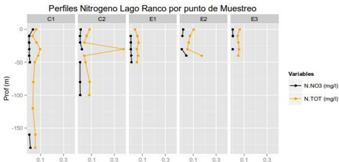
Figura 70. Perfiles de compuestos nitrogenados (N-NO 3 en mg/L y NT en mg/L) de la columna de agua en los centros analizados en el lago Ranco (E1 corresponde a la concesión 100978, y E2 a 101955).
