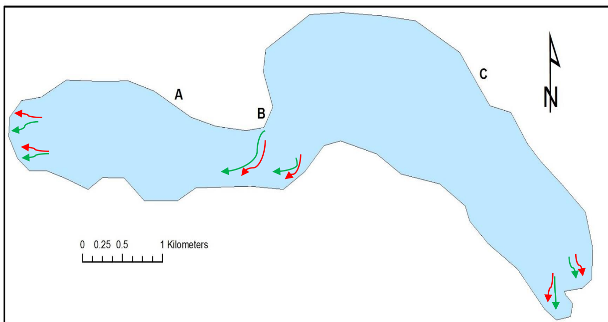
Figura 58. Mediciones de correntometría en el tramo A y B del lago Tarahuín. Color verde= correntometría de superficie, color rojo= correntometría de profundidad.
