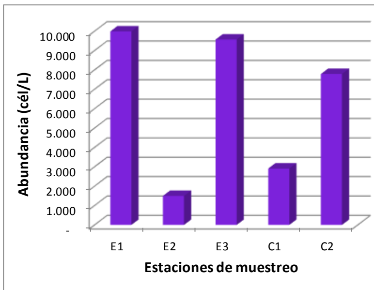
Figura 63. Abundancia fitoplanctónica (cél/L) en las estaciones de muestreo del lago Cucao, durante el invierno de 2014.
