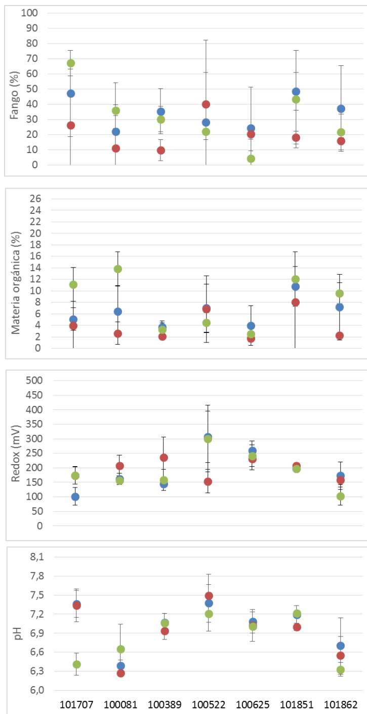
Figura 84. Lago Rupanco: valores promedio y desviaci3n estandar de fango (%), materia orgánica (%), redox (mV) y pH en sedimentos para las diferentes estaciones de muestreo
