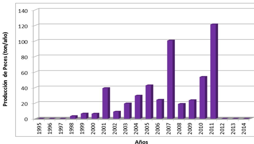
Figura 133. Producción histórica de peces (ton/año) en el lago Ranco.
