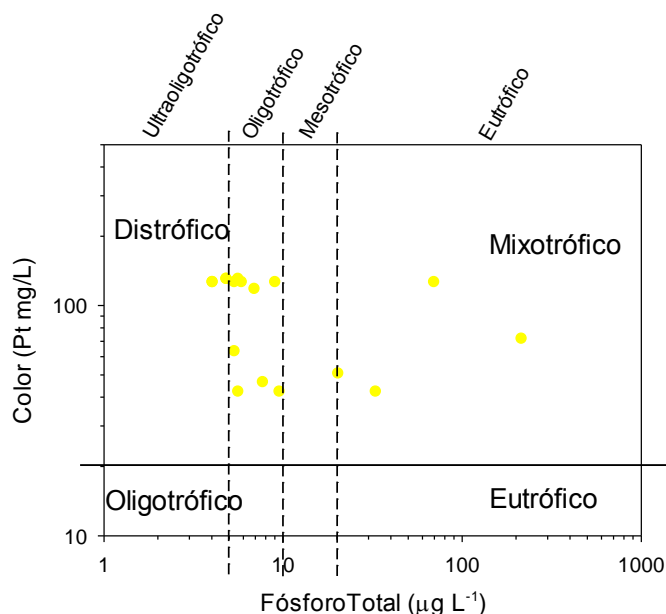
Figura 124. Clasificación paradigma nutriente - color para caracterizar lago Cucao.
