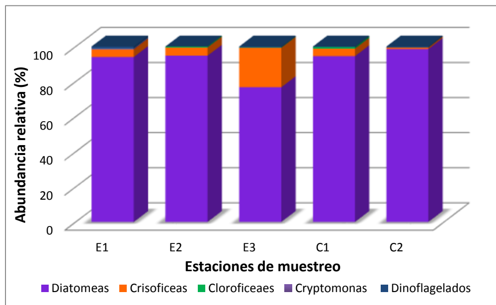
Figura 71. Abundancia relativa (%) en las estaciones de muestreo del lago Ranco, durante la primavera de 2014.
