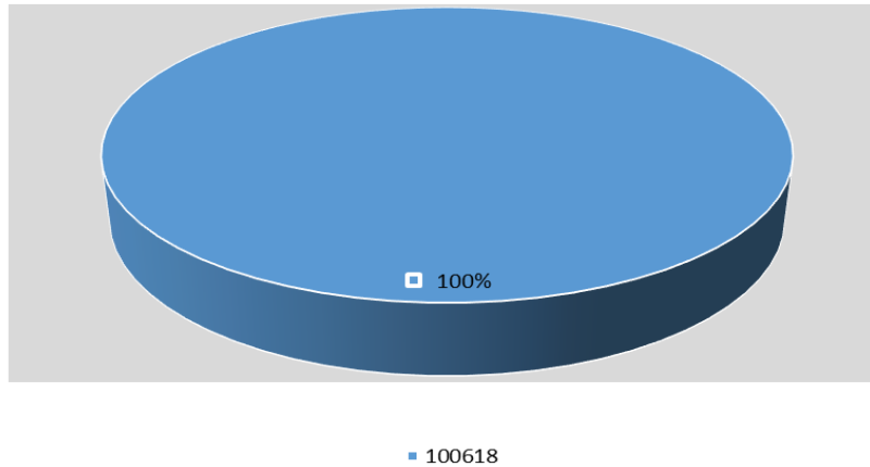
Figura 126. Producción histórica (%) por centro de cultivo en el lago Cucao.
