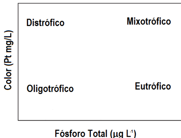
Figura 11. Modelo conceptual de paradigma nutriente – color, extraído y modificado desde Williamson et al. (1999) y Webster et al. (2008).
