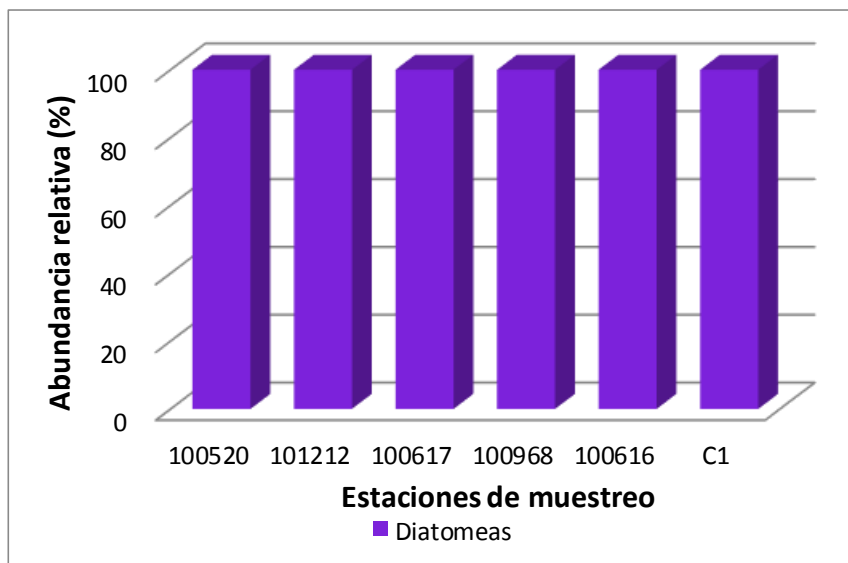
Figura 44. Abundancia relativa (%) en las estaciones de muestreo del lago Huillenco, durante el invierno de 2014.
