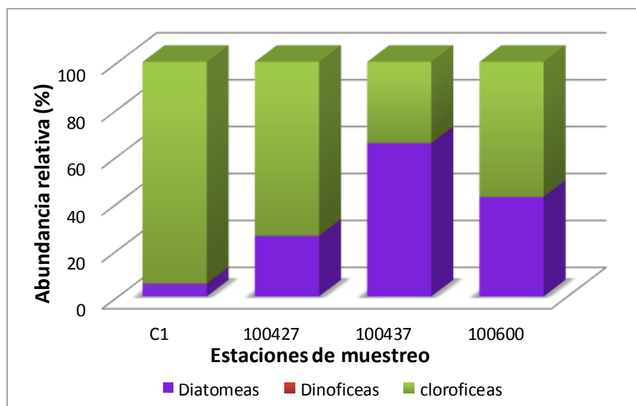
Figura 35. Abundancia relativa (%) en las estaciones de muestreo del lago Natri, durante el invierno de 2014.
