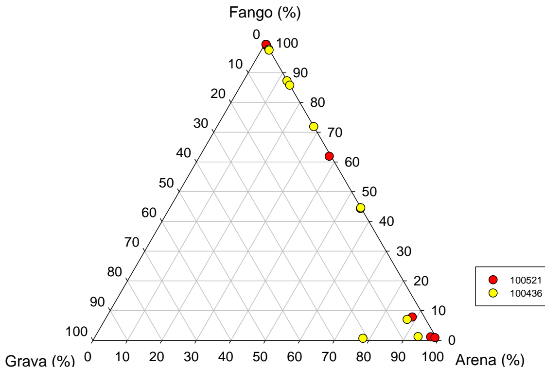
Figura 56. Gráfico de triángulo para clasificación de textura del lago Tarahuín (% fango, % arena y % grava).
