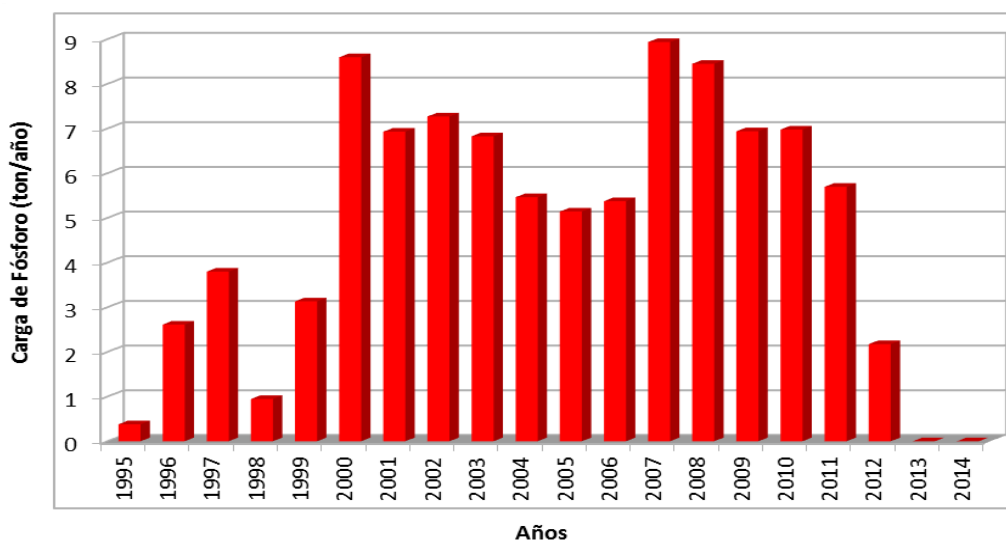
Figura 122. Aporte de PT (ton/a3o) desde centros de cultivo en el lago Tarahu3n.
