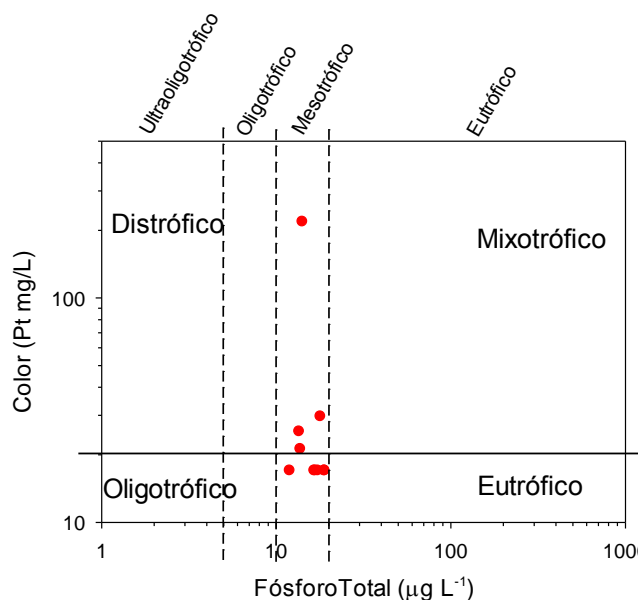
Figura 119. Clasificaci3n paradigma nutriente - color para caracterizar lago Tarahuín.
