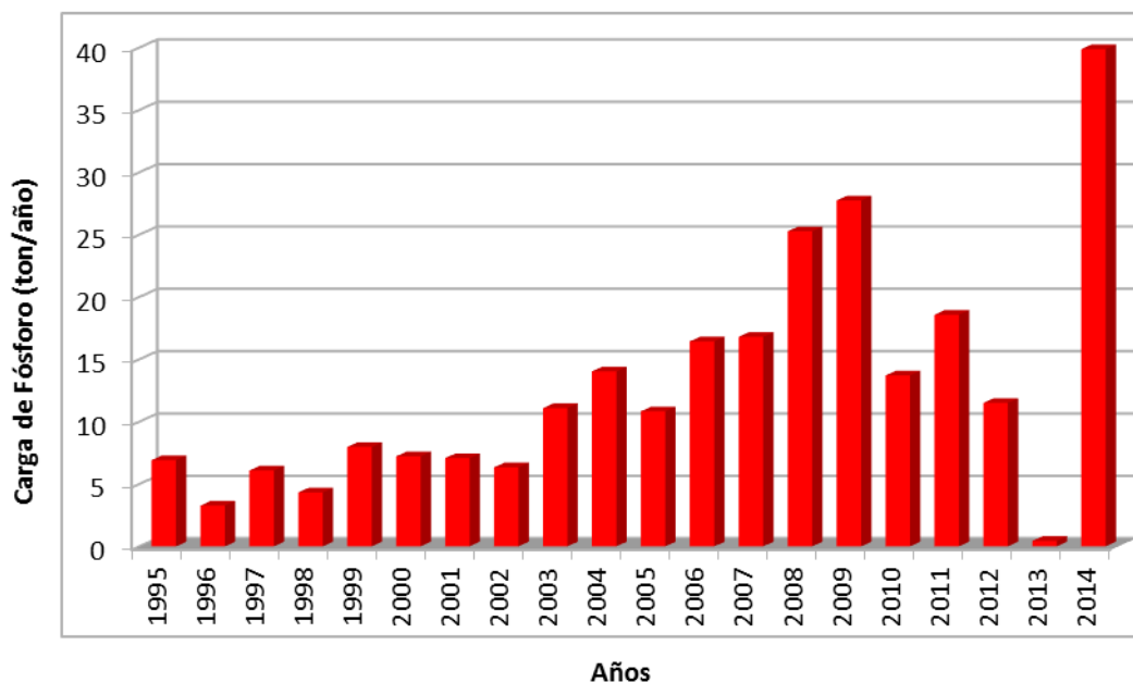
Figura 107. Aporte de PT (ton/a3o) desde centros de cultivo en el lago Chapo.
