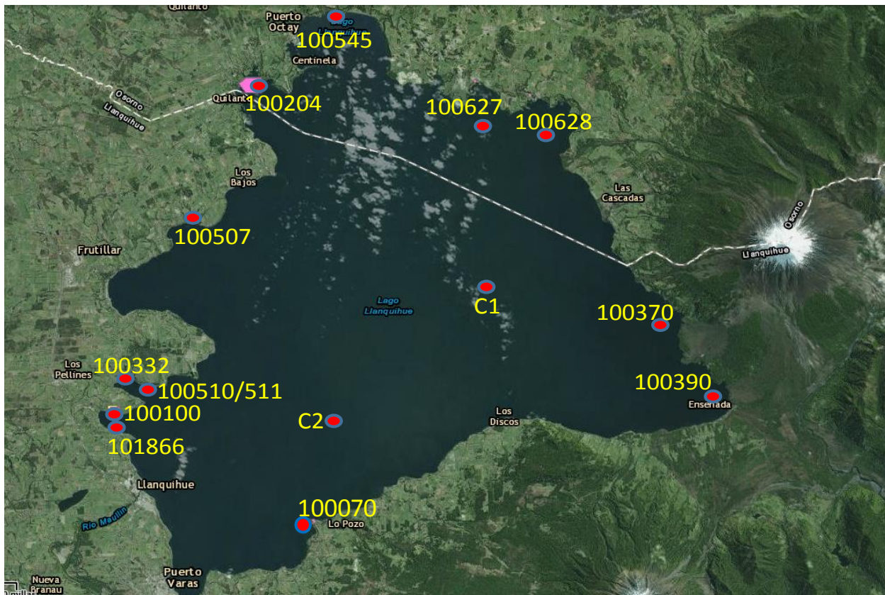
Figura 5. Estaciones de muestreo en lago Llanquihue (en la figura se identifican 13 c3digos pertenecientes a concesiones de acuicultura, en donde se tomaron las muestras: 101866, 100100, 100510/511, 100332, 100507, 100204, 100545, 100627, 100628, 100370, 100390, 100070; adem3s de dos sitios control de m3xima profundidad, C1 y C2).
