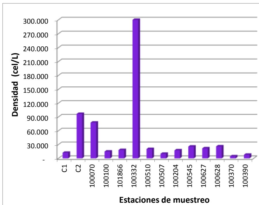
Figura 18. Abundancia fitoplanctónica (cél/L) en las estaciones de muestreo del lago Llanquihue, durante el otoño de 2014.
