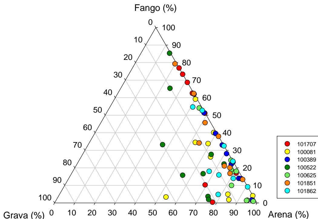
Figura 83. Lago Rupanco: Gráfico de triángulo para clasificación de textura (% fango, % arena y % grava).
