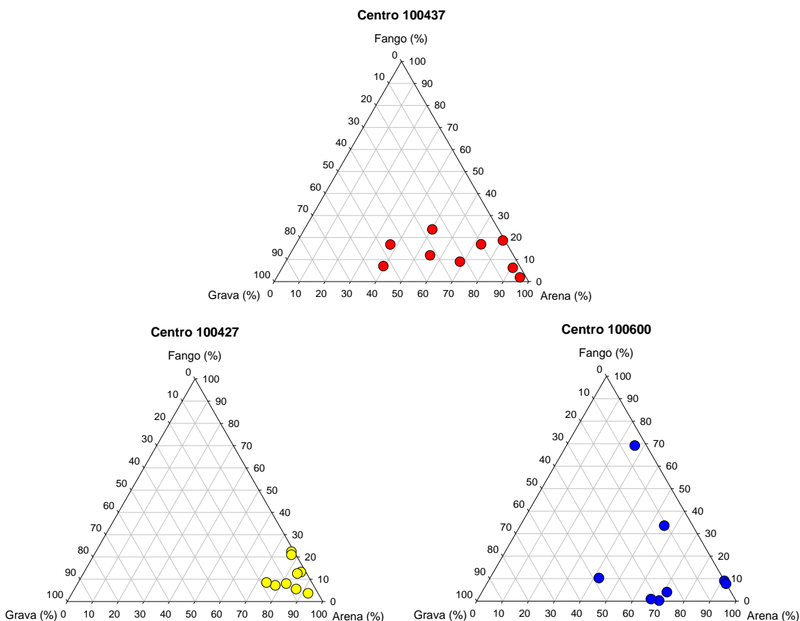
Figura 37. Lago Natri: Fracciones texturales (% fango, % arena y % grava) representadas en un gráfico de triángulo para cada centro.
