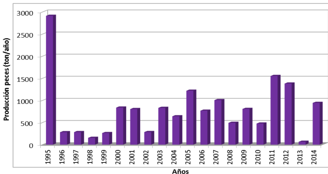
Figura 110. Producción histórica de peces (ton/año) en el lago Natri.
