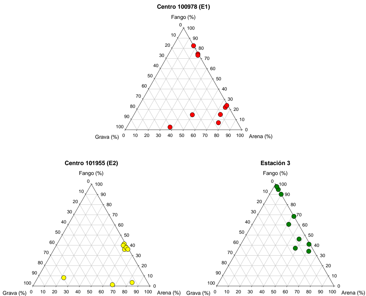
Figura 73. Lago Ranco: Fracciones texturales (% fango, % arena y % grava) representadas en un gr3fico de tri3ngulo para cada centro.
