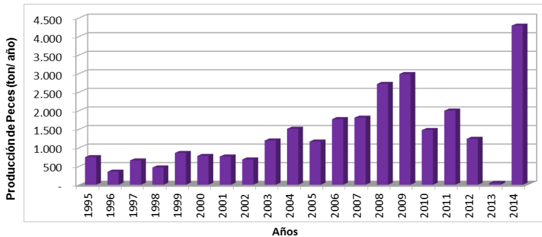
Figura 105. Producción histórica de peces (ton/año) en el lago Chapo.
