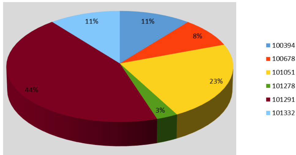
Figura 106. Producción histórica (%) por centro de cultivo en el lago Chapo.
