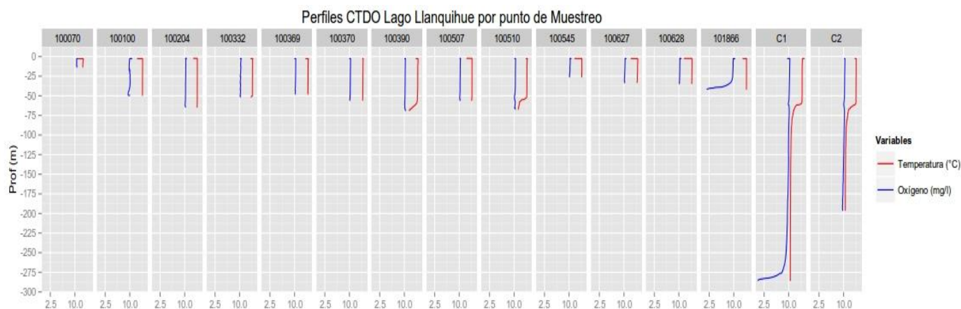
Figura 14. Perfiles físico-químicos (oxígeno en mg/L y temperatura en °C) de la columna de agua de los centros analizados en el lago Llanquihue.
