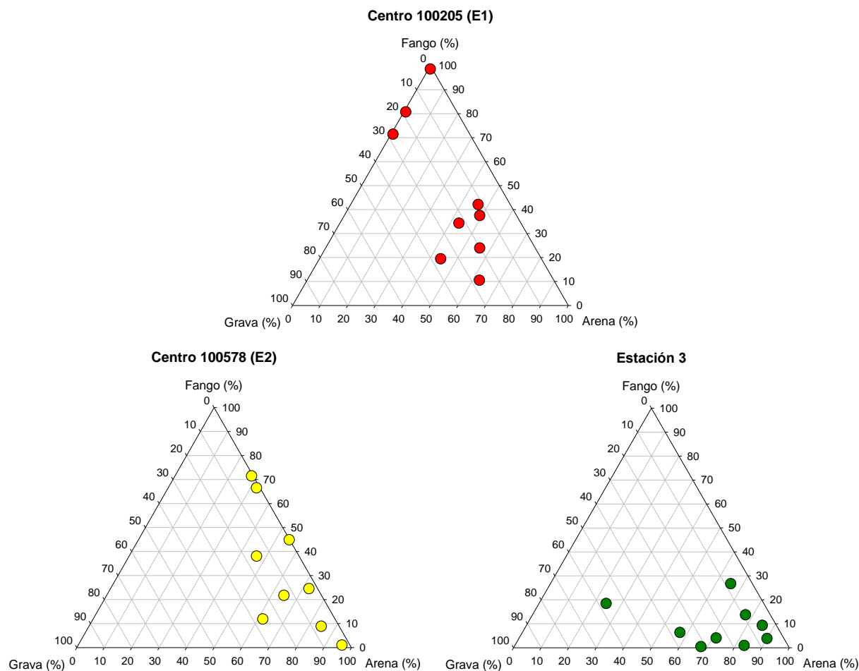
Figura 91. Lago Puyehue: Fracciones texturales (% fango, % arena y % grava) representadas en un gráfico de triángulo para cada centro.
