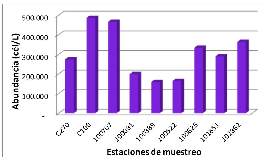
Figura 81. Abundancia fitoplanct3nica (c3l/L) en las estaciones de muestreo del lago Rupanco, durante la primavera de 2014.
