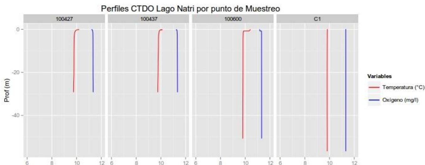
Figura 32. Perfiles físico-químicos (oxígeno en mg/L y temperatura en °C) de la columna de agua de los centros analizados en el lago Natri.
