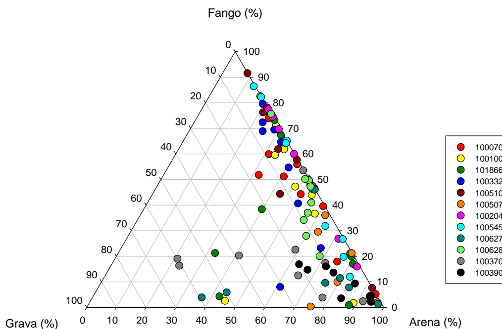
Figura 20. Lago Llanquihue: Gráfico triangular para la clasificación de textura de los sedimentos del lago Llanquihue (% fango, % arena y % grava).
