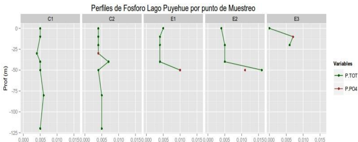
Figura 87. Perfiles de ortofosfato ( P-PO_4 en mg/L) y fósforo total (PT en mg/L) de la columna de agua de los centros analizados en el lago Puyehue.
