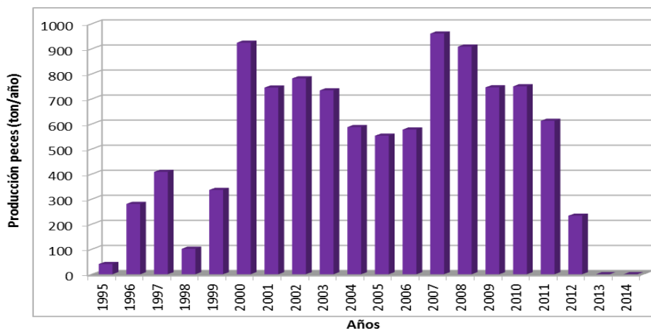
Figura 120. Producci3n hist3rica de peces (ton/a3o) en el lago Tarahuín.
