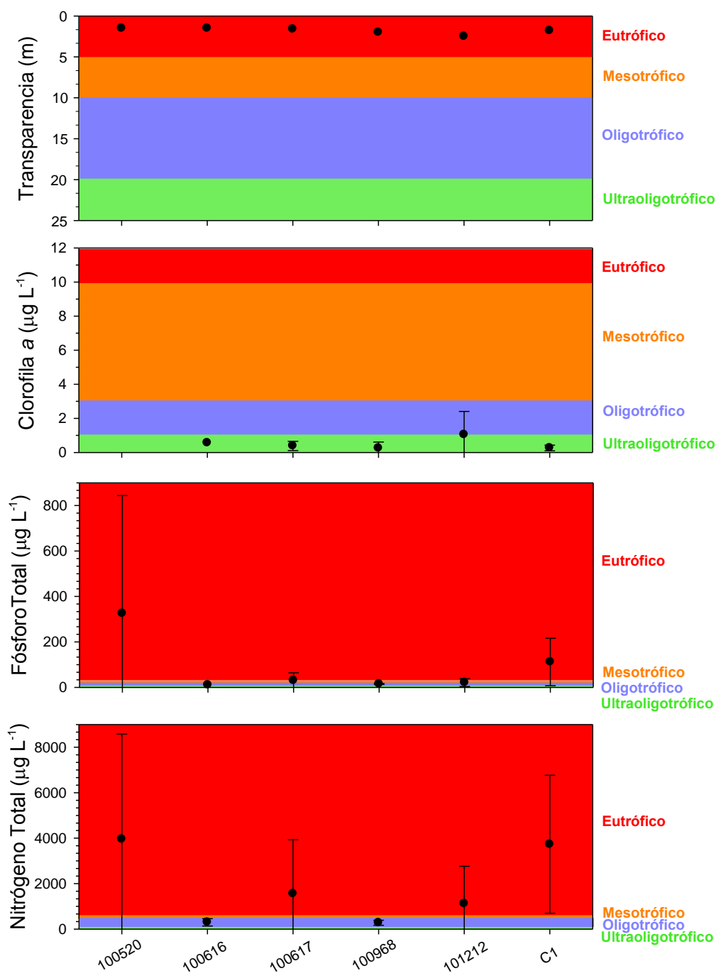
Figura 113. Indicadores tróficos: Transparencia (m), clorofila a ( \mu\text{g L}^{-1} ), fósforo total ( \mu\text{g L}^{-1} ) y nitrógeno total ( \mu\text{g L}^{-1} ) en lago Huillínco.
