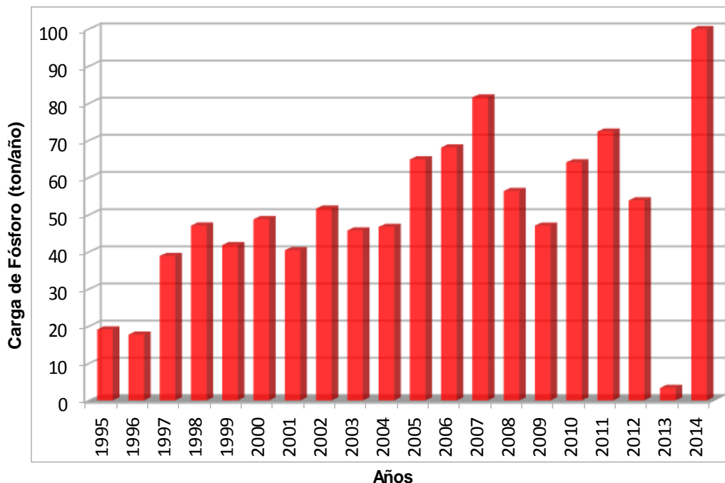
Figura 101. Aporte de PT (ton/a3o) desde centros de cultivo en el lago Llanquihue.
