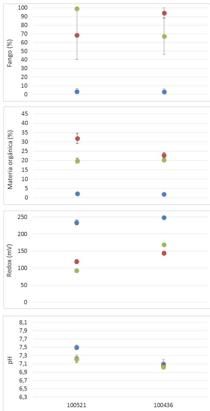
Figura 57. Lago Tarahuín: valores promedio y desviación estándar de fango (%), materia orgánica (%), redox (mV) y pH en sedimentos para las diferentes estaciones de muestreo.
