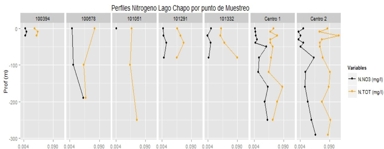
Figura 25. Perfiles compuestos nitrogenados (N-NO 3 en mg/L, NT en mg/L) en los centros analizados del lago Chapo (---N-NO 3 ; ---NT).
