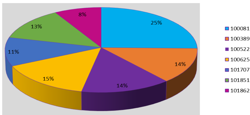
Figura 130. Producci3n hist3rica (%) por centro de cultivo en el lago Rupanco.
