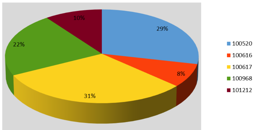
Figura 116. Producción histórica (%) por centro de cultivo en el lago Huillín.
