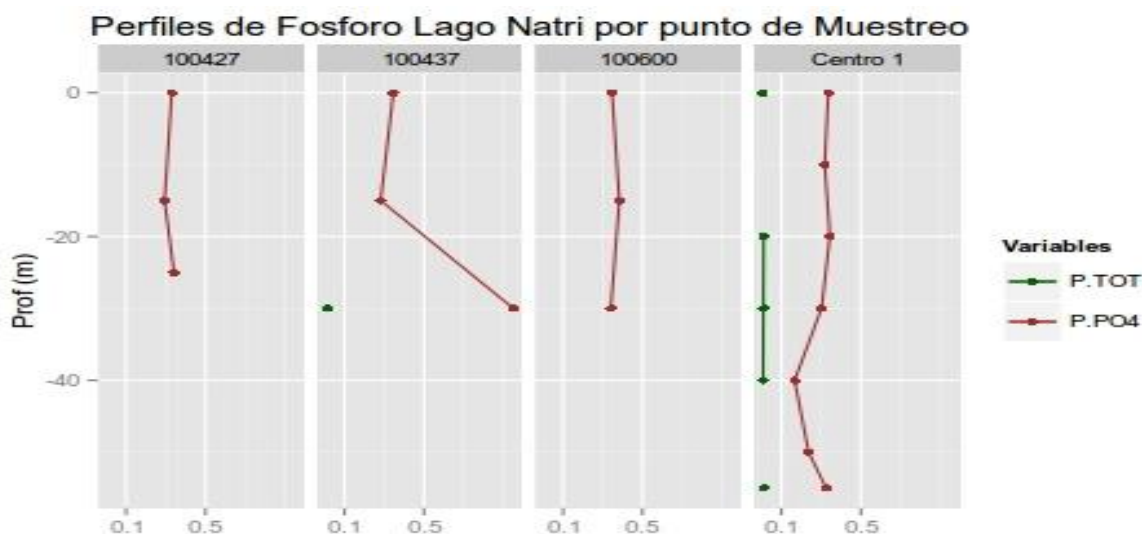
Figura 33. Perfiles de ortofosfato (P-PO 4 en mg/L) y f3sforo total (PT en mg/L) de la columna de agua de los centros analizados en el lago Natri.
