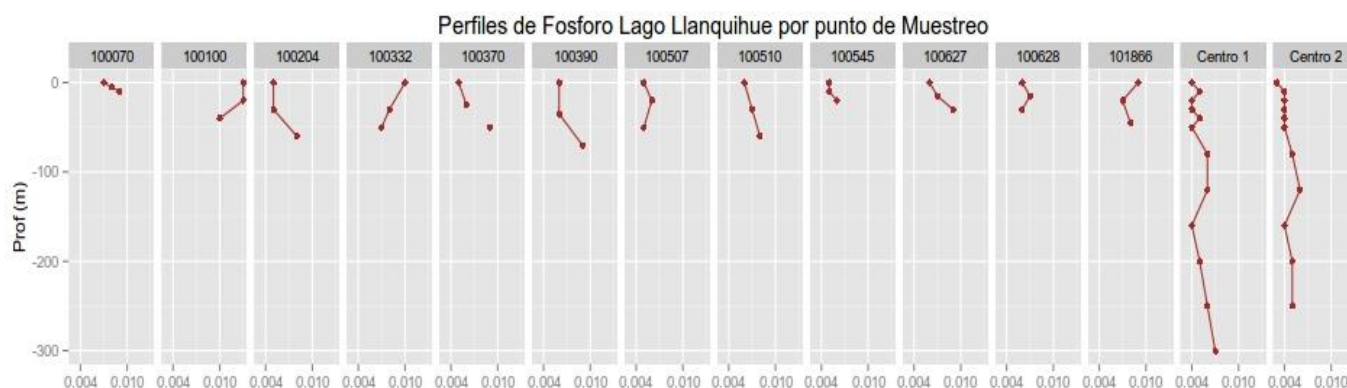
Figura 15. Perfiles de f3sforo total (PT en mg/L) de la columna de agua de los centros analizados en el lago Llanquihue (PT).
