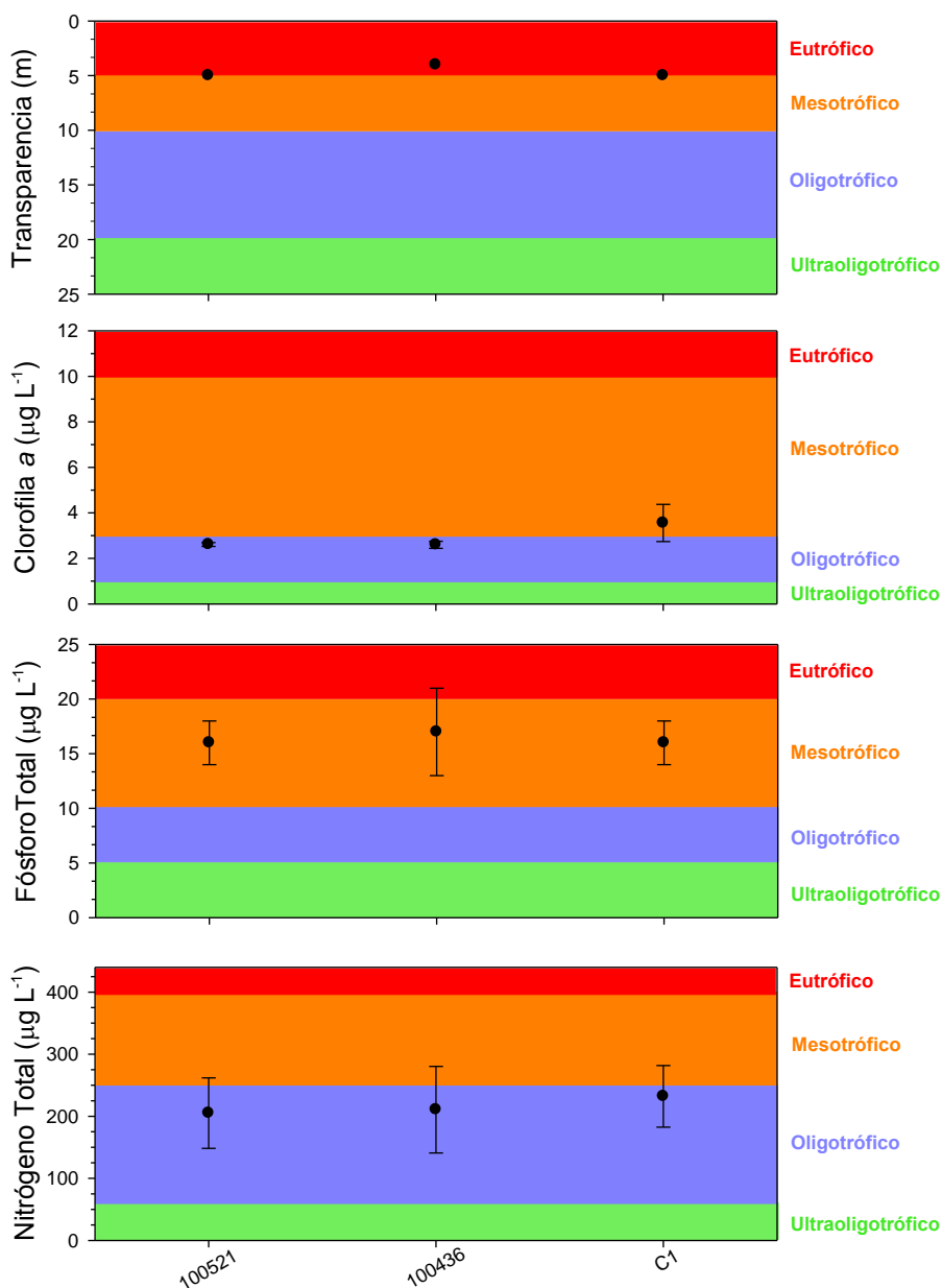
Figura 118. Indicadores tróficos: Transparencia (m), clorofila a ( \mu\text{g L}^{-1} ), fósforo total ( \mu\text{g L}^{-1} ) y nitrógeno total ( \mu\text{g L}^{-1} ) en lago Tarahuín.
