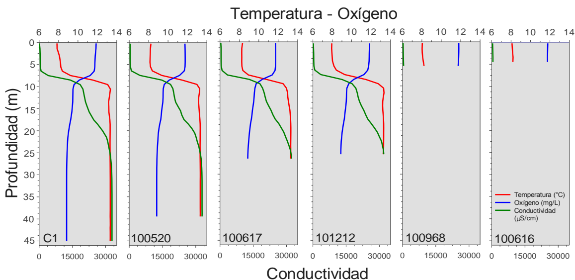
Figura 41. Perfiles físico-químicos (conductividad en mS/cm, oxígeno en mg/L, y temperatura en °C) de la columna de agua de los centros analizados del lago Huillinco.
