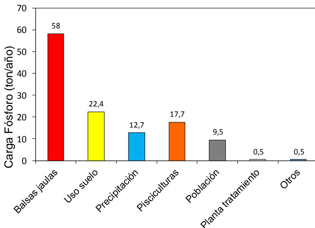
Figura 102. Carga de f3sforo total (ton/a3o) seg3n actividad.
