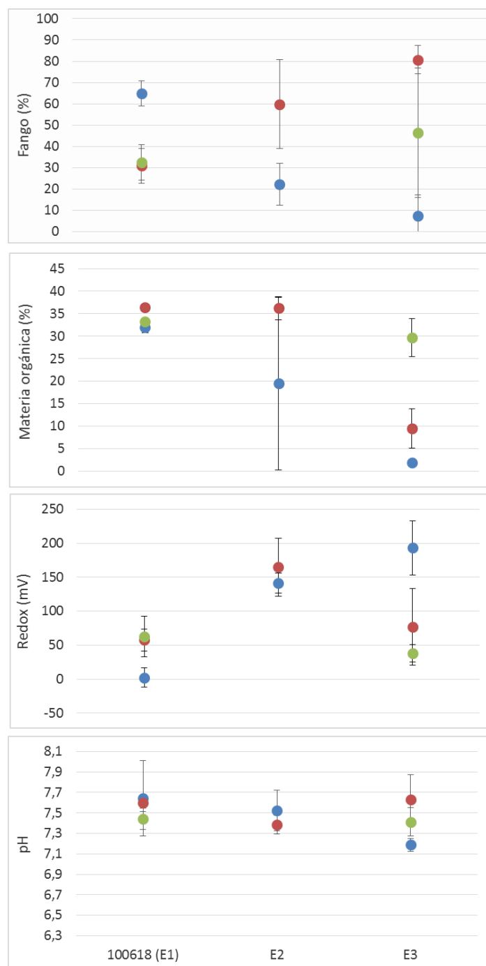
Figura 66. Lago Cucao: valores promedio y desviación estándar de fango (%), materia orgánica (%), redox (mV) y pH en sedimentos para las diferentes estaciones de muestreo. E1 corresponde a la concesión 100618.
