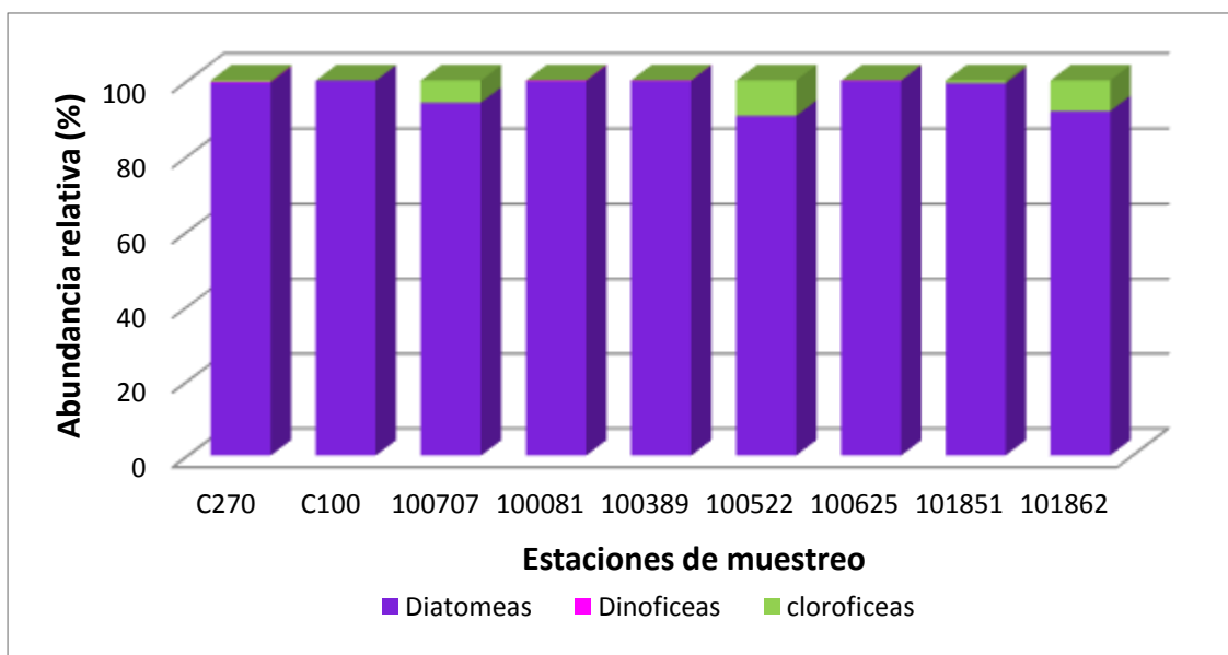
Figura 80. Abundancia relativa (%) en las estaciones de muestreo del lago Rupanco, durante la primavera de 2014.
