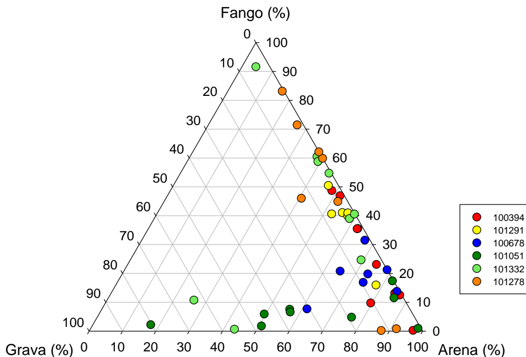
Figura 29. Lago Chapo: Gráfico de triángulo para clasificación de textura (% fango, % arena y % grava).
