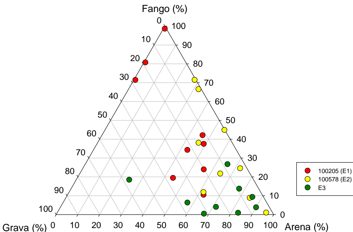
Figura 92. Lago Puyehue: Gráfico de triángulo para clasificación de textura del lago Puyehue (% fango, % arena y % grava).
