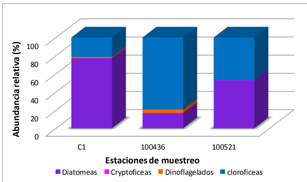
Figura 53. Abundancia relativa (%) en las estaciones de muestreo del lago Tarahuín, durante el invierno de 2014.
