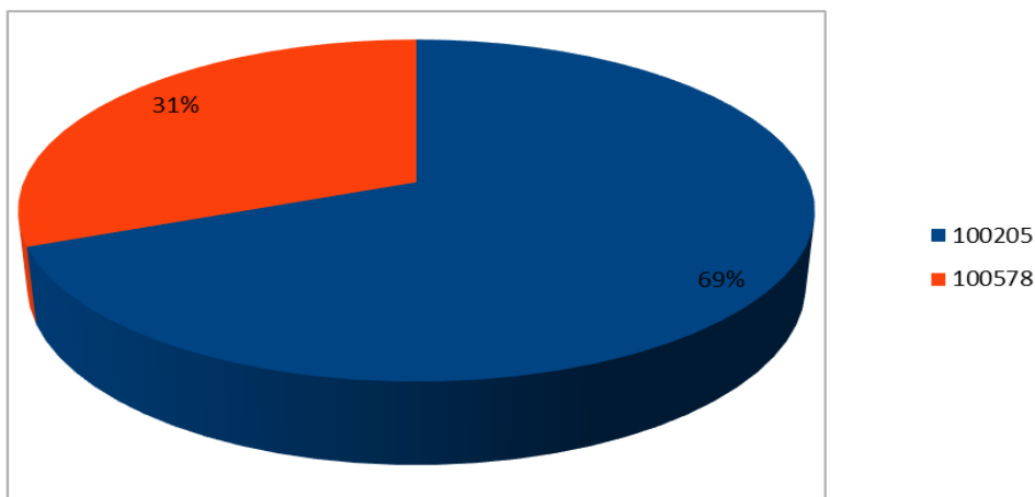
Figura 138. Producci3n hist3rica (%) por centro de cultivo en el lago Puyehue.
