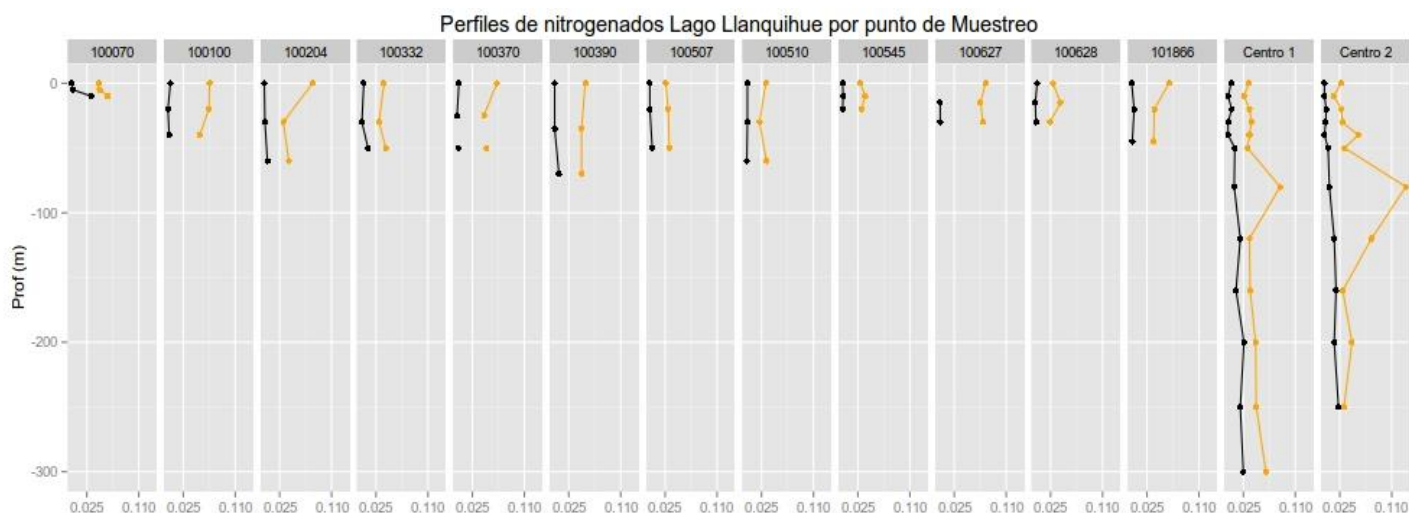
Figura 16. Perfiles de compuestos nitrogenados ( \text{N-NO}_3 en mg/L y NT en mg/L) de la columna de agua de los centros analizados en el lago Llanquihue (--- \text{N-NO}_3 , ---NT).
