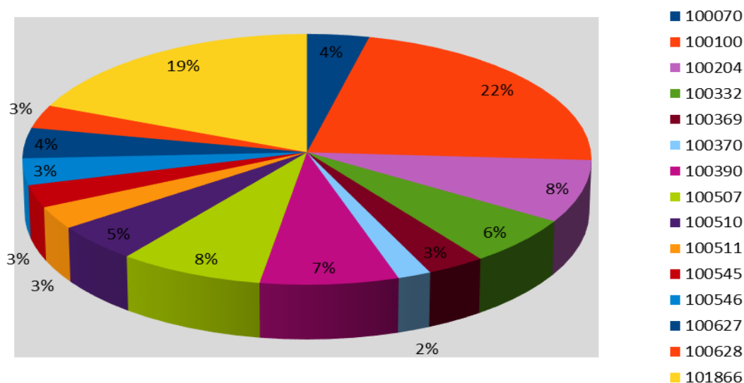
Figura 100. Producción histórica (%) por centro de cultivo en el lago Llanquihue.
