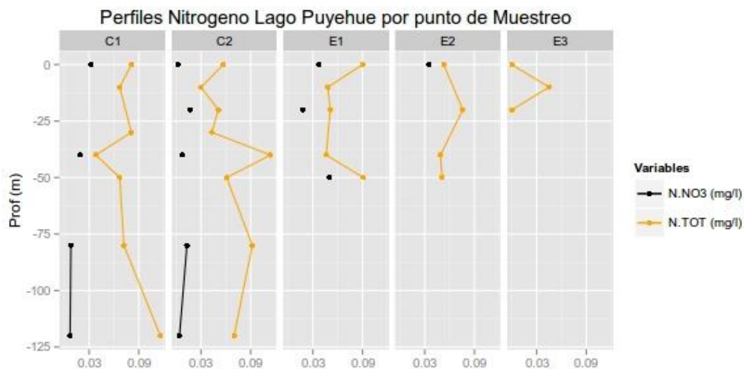
Figura 88. Perfiles de compuestos nitrogenados ( N-NO_3 en mg/L y NT en mg/L) de la columna de agua de los centros analizados en el lago Puyehue.
