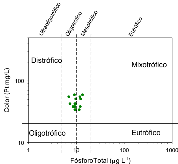
Figura 109. Clasificaci3n paradigma nutriente - color para caracterizar lago Natri.
