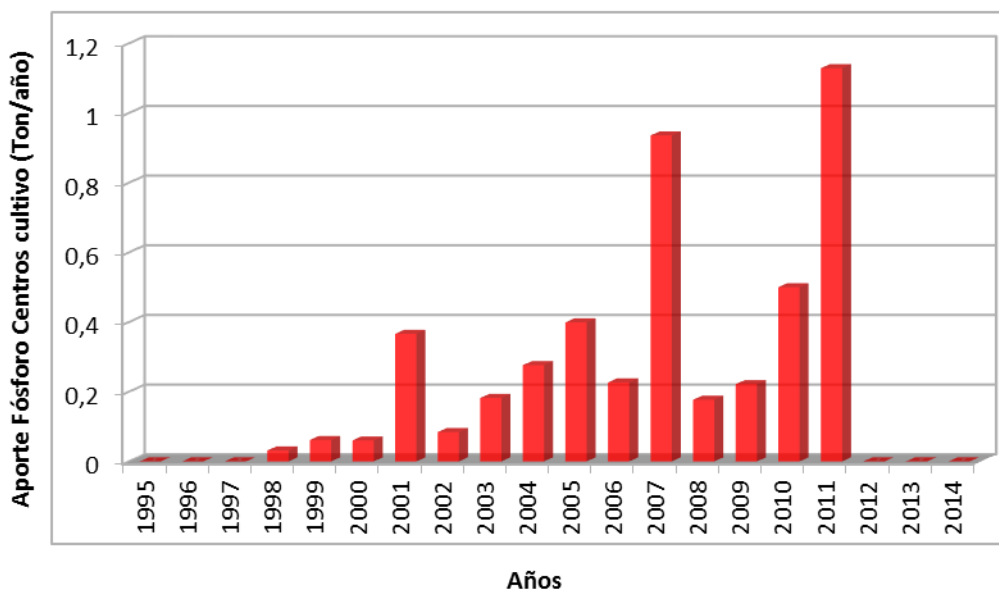
Figura 135. Aporte de PT (ton/año) desde centros de cultivo en el lago Ranco.
