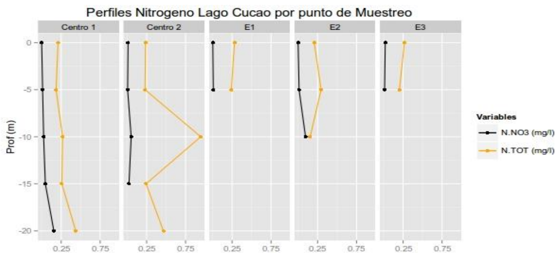
Figura 61. Perfiles de compuestos nitrogenados (N-NO 3 en mg/L y NT en mg/L) de la columna de agua en los centros analizados del lago Cucao (E1 corresponde a la concesión 100618).
