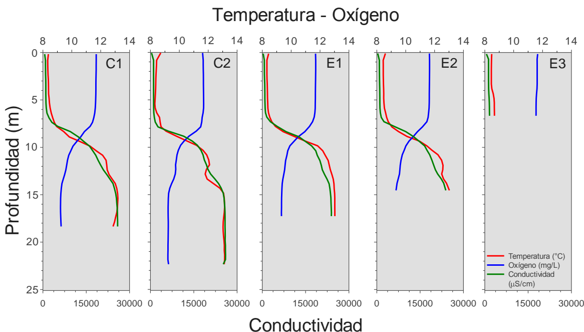
Figura 59. Perfiles físico-químicos (conductividad en mS/cm, oxígeno en mg/L y temperatura en °C) de la columna de agua en las estaciones analizadas del lago Cucao (E1 corresponde a la concesión 100618).
