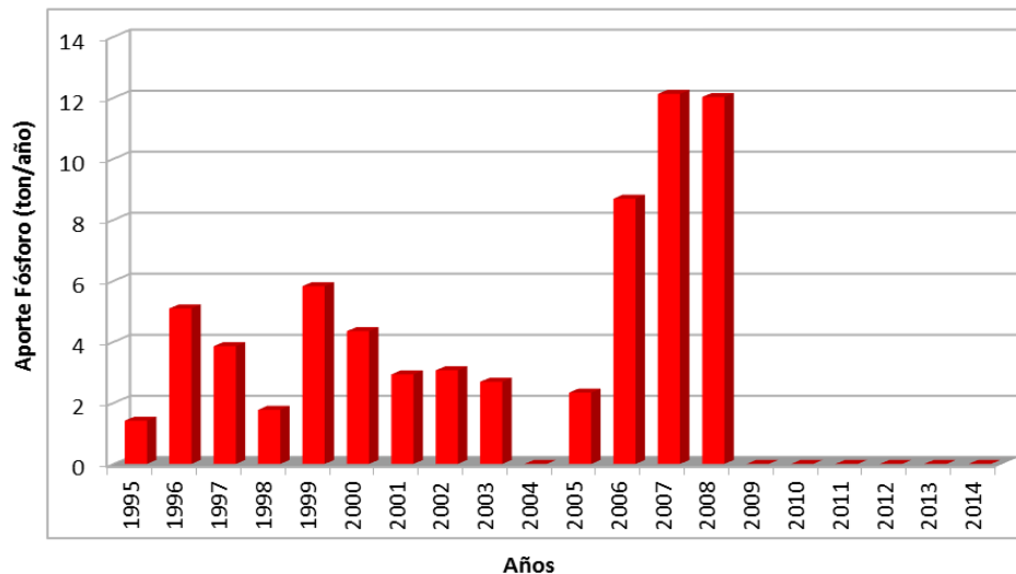
Figura 127. Aporte de PT (ton/año) desde centros de cultivo en el lago Cucao.
