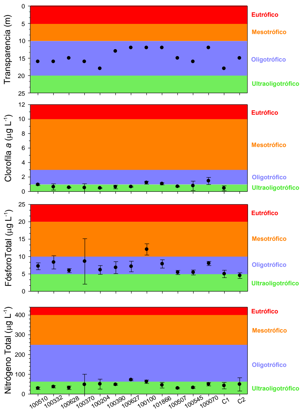
Figura 95. Indicadores tróficos: Transparencia (m), clorofila a ( \mu\text{g L}^{-1} ), fósforo total ( \mu\text{g L}^{-1} ) y nitrógeno total ( \mu\text{g L}^{-1} ) en lago Llanquihue.
