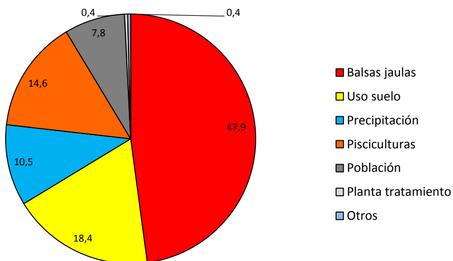
Figura 103. Contribuci3n de f3sforo total (%) seg3n actividad.
