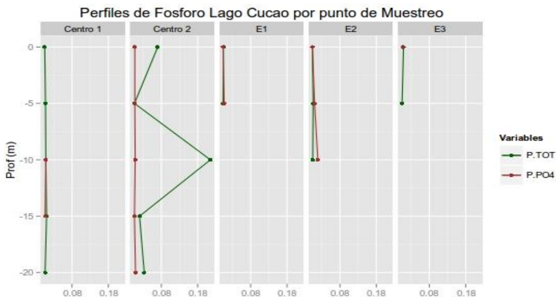
Figura 60. Perfiles de ortofosfato (P-PO 4 en mg/L) y fósforo total (PT en mg/L) en la columna de agua en los centros analizados del lago Cucao (E1 corresponde a la concesión 100618).
