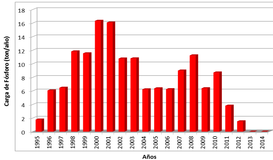
Figura 117. Aporte de PT (ton/año) desde centros de cultivo en el lago Huillínco.
