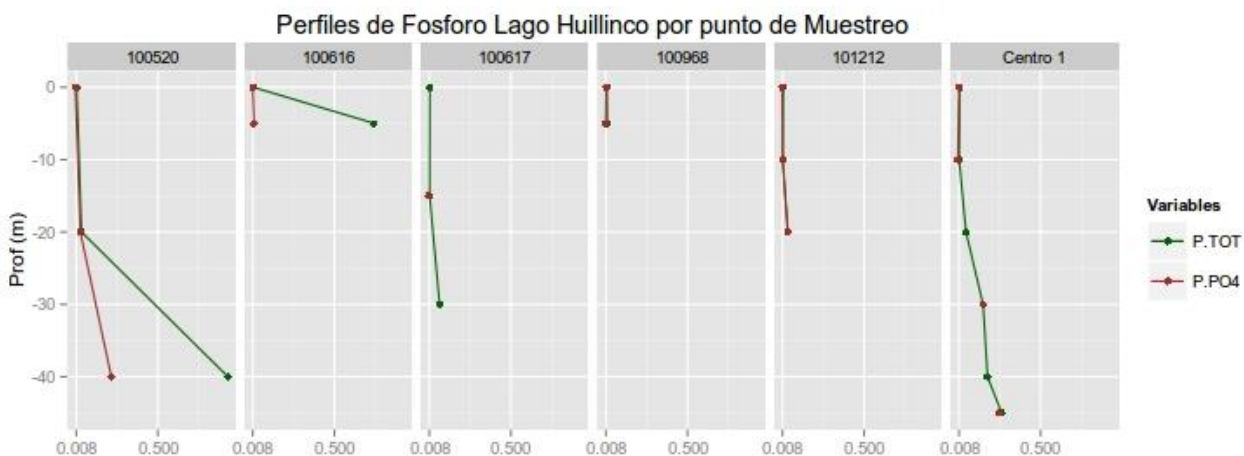
Figura 42. Perfiles de ortofosfato ( P-PO_4 en mg/L) y fósforo total (PT en mg/L) en los centros analizados del lago Huillanco.
