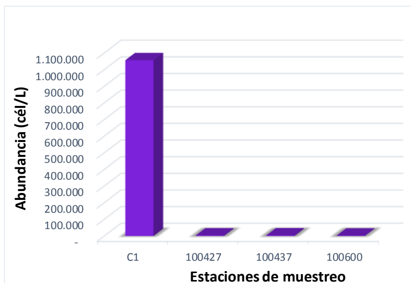
Figura 36. Abundancia fitoplanct3nica (c3l/L) en las estaciones de muestreo del lago Natri, durante el invierno de 2014.
