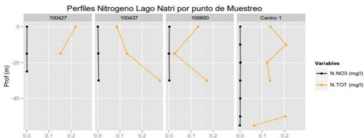
Figura 34. Perfiles de compuestos nitrogenados (N-NO 3 en mg/L y NT en mg/L) de la columna de agua de los centros analizados en el lago Natri.
