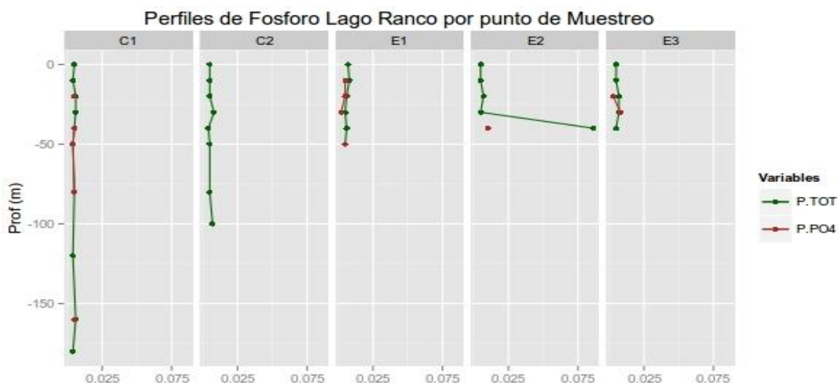
Figura 69. Perfiles de ortofosfato (P-PO 4 en mg/L) y fósforo total (PT en mg/L) de la columna de agua en los centros analizados en el lago Ranco (E1 corresponde a la concesión 100978, y E2 a 101955).
