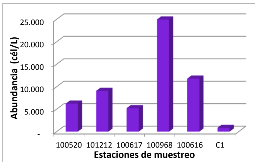
Figura 45. Abundancia fitoplanctónica (cél/L) en las estaciones de muestreo del lago Huillínco, durante el invierno de 2014.
