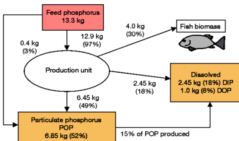
Figura 12. Flujos de P (kg PT/ton peces producidos) estimados para la salmonicultura (figura extraída del Informe final de la primera parte del proyecto).
