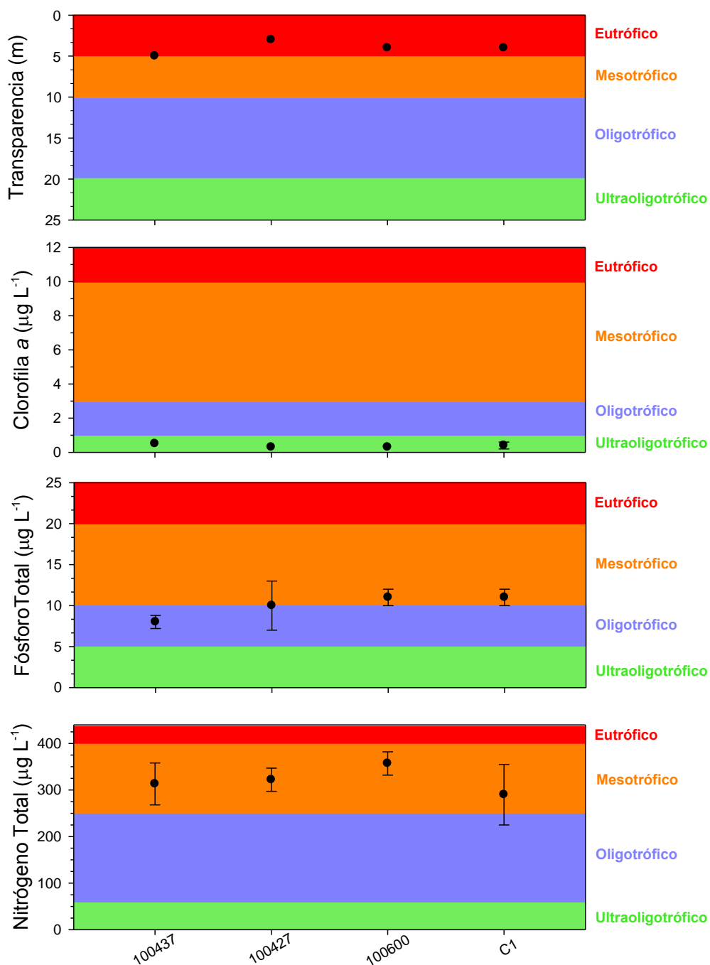
Figura 108. Indicadores tr3ficos: Transparencia (m), clorofila a ( \mu\text{g L}^{-1} ), f3sforo total ( \mu\text{g L}^{-1} ) y nitr3geno total ( \mu\text{g L}^{-1} ) en lago Natri.
