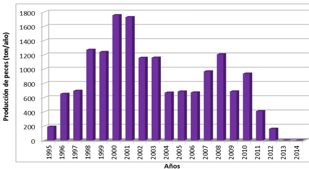
Figura 115. Producción histórica de peces (ton/año) en el lago Huillín.
