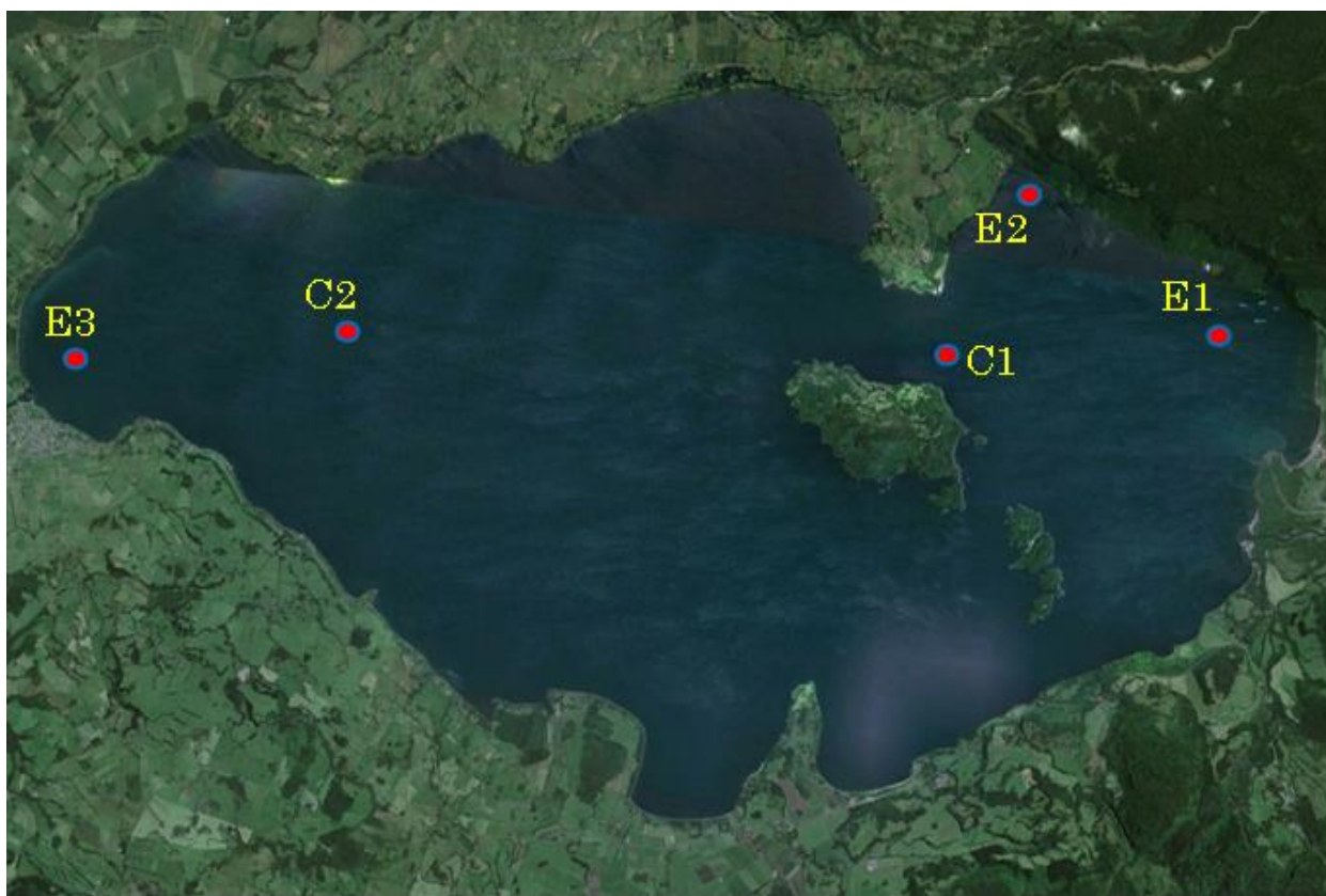
Figura 3. Estaciones de muestreo en lago Puyehue (E1 y E2 corresponden a estaciones de muestreo en bahías con concesiones de acuicultura autorizadas, 100205 y 100578 respectivamente, mientras que E3 a la Bahía cercana al poblado Entrelagos. C2 y C1 corresponden a sitios control de máxima profundidad del lago).
