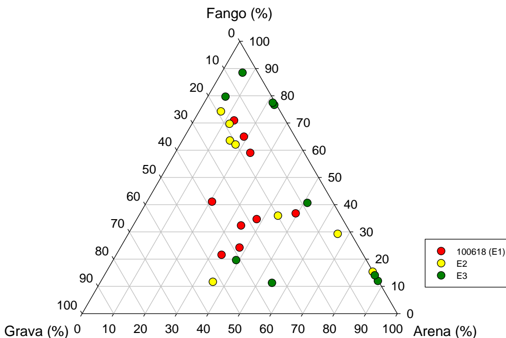
Figura 65. Lago Cucao: Gráfico de triángulo para clasificación de textura (% fango, % arena y % grava).
