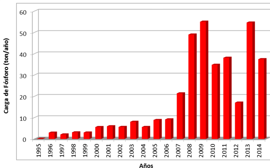
Figura 139. Aporte de PT (ton/a3o) desde centros de cultivo en el lago Puyehue.
