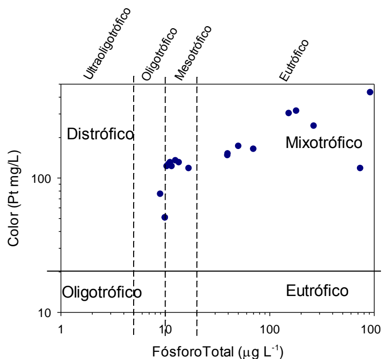
Figura 114. Clasificaci3n paradigma nutriente - color para caracterizar lago Huillenco.
