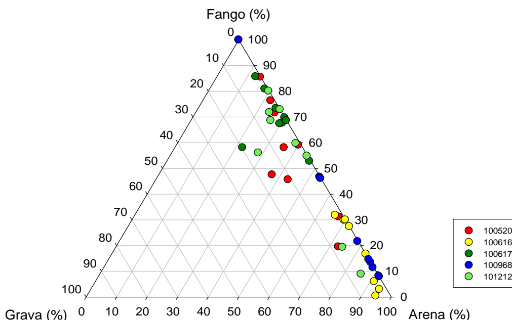
Figura 47. Lago Huillinco: Gráfico de triángulo para clasificación de textura (% fango, % arena y % grava).
