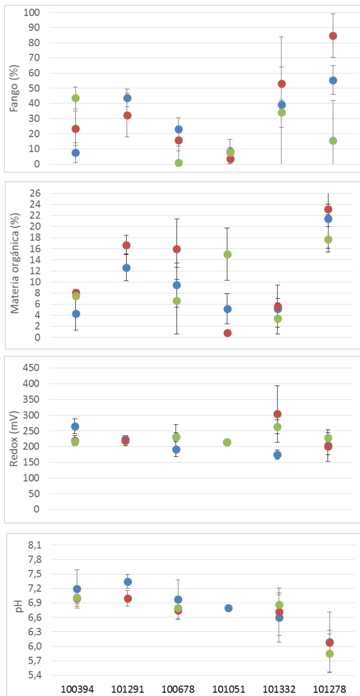
Figura 30. Lago Chapo: valores promedio y desviación estándar de fango (%), materia orgánica (%), redox (mV) y pH en sedimentos para las diferentes estaciones de muestreo.
