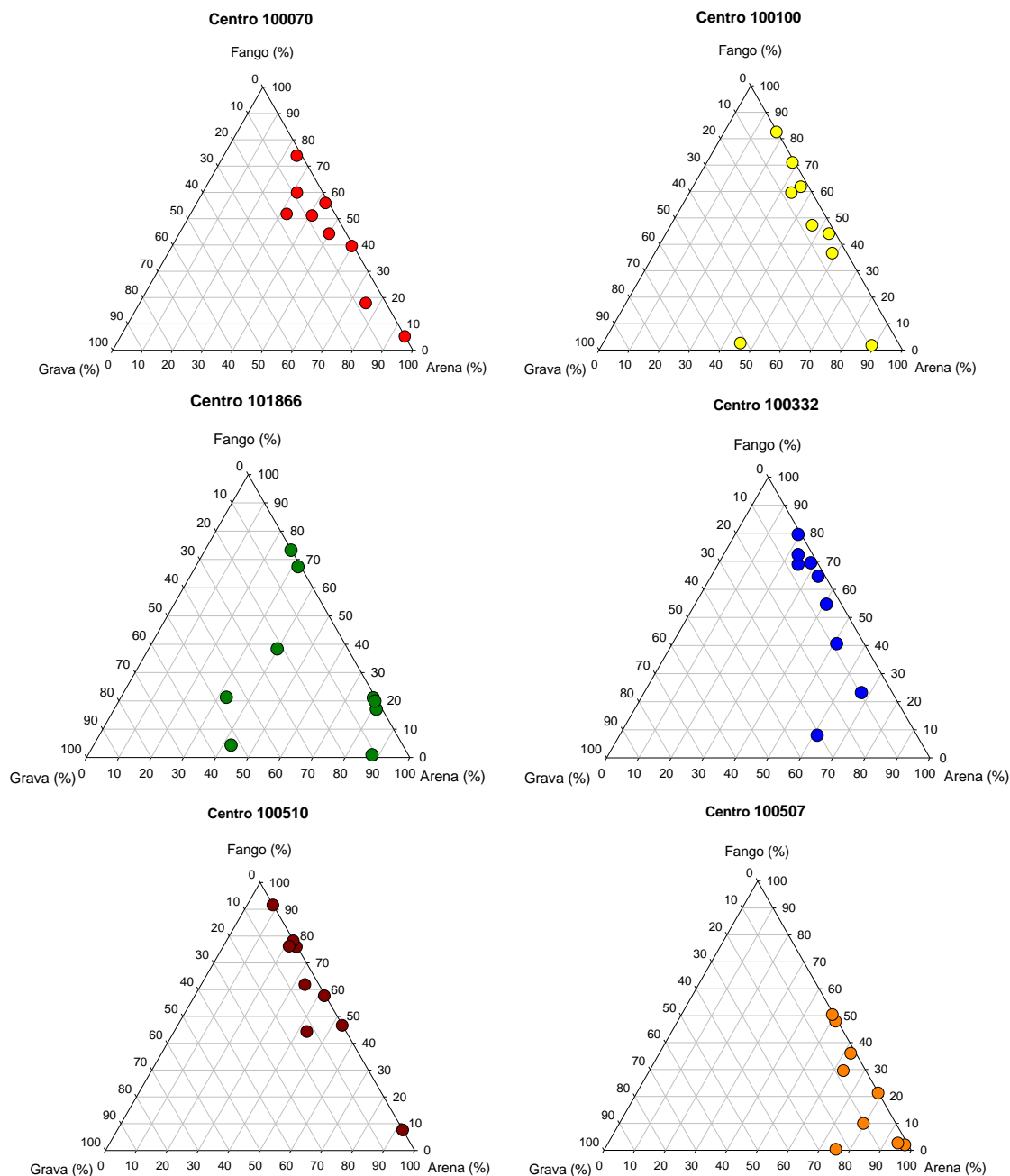
Figura 19. Lago Llanquihue: Fracciones texturales (% fango, % arena y % grava) representadas en un gráfico de triángulo para cada centro. Maitén A (100510), Maitén C (100332), Bahía Cox (100628), Bahía Ensenada (100370), Bahía Rincones (100204), Bahía Volcán (100390), Monte Alegre (100627), Puerto Phillipi I (100100), Puerto Phillipi 2 (101866), Playa Maqui (100507), Puerto Octay (100545) y Puerto Rosales (1000070).
