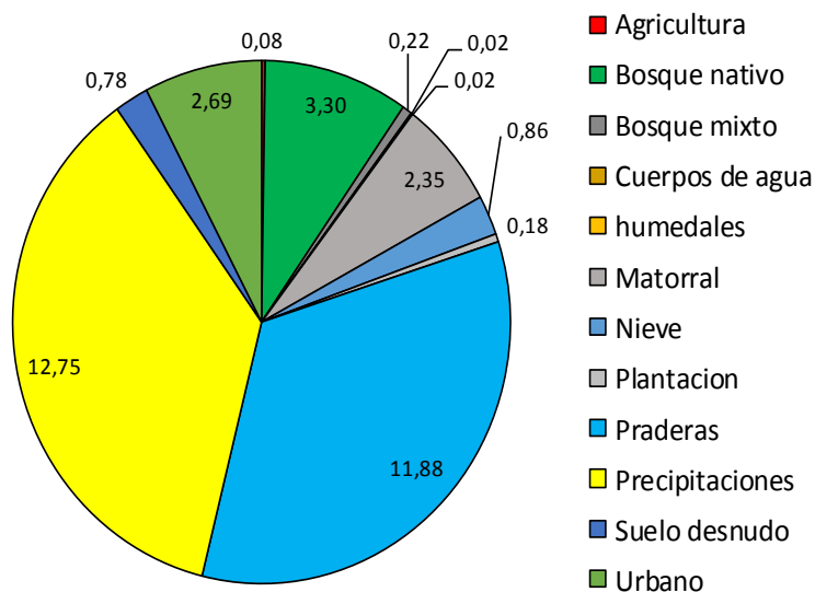
Figura 98. Aporte de f3sforo total (ton/a3o) seg3n uso de suelo.
