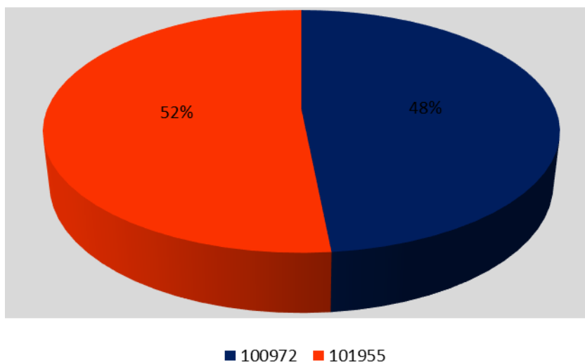
Figura 134. Producción histórica (%) por centro de cultivo en el lago Ranco.
