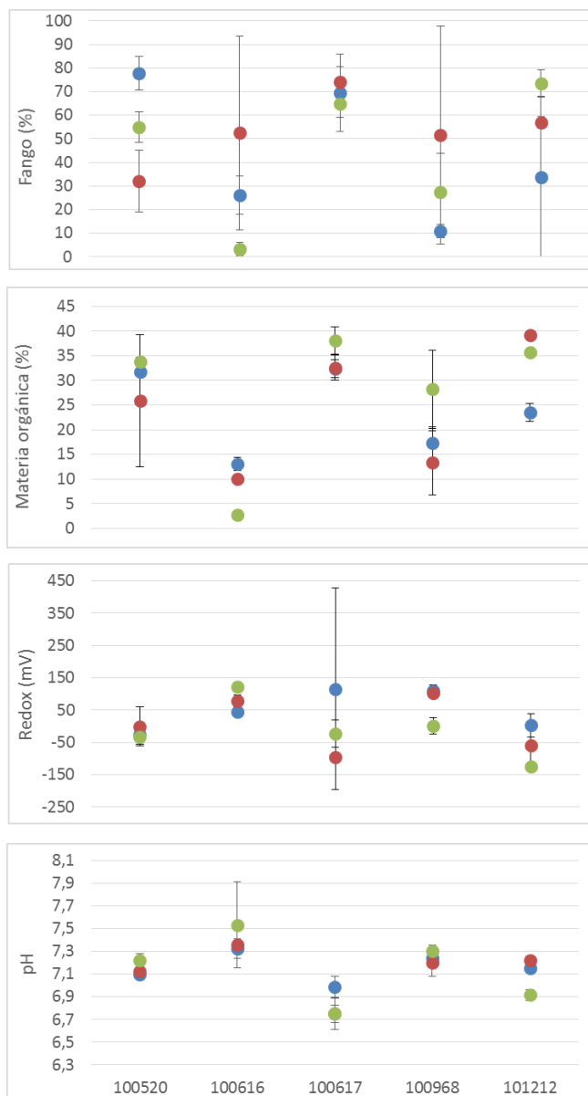
Figura 48. Lago Huillincó: valores promedio y desviación estándar de fango (%), materia orgánica (%), redox (mV) y pH en sedimentos para las diferentes estaciones de muestreo.
