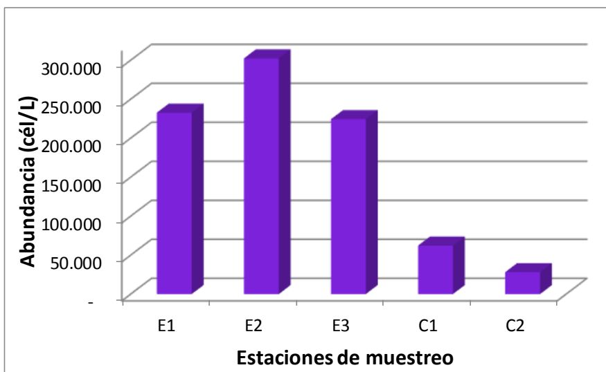
Figura 72. Abundancia fitoplanctónica (cél/L) en las estaciones de muestreo del lago Ranco, durante la primavera de 2014.
