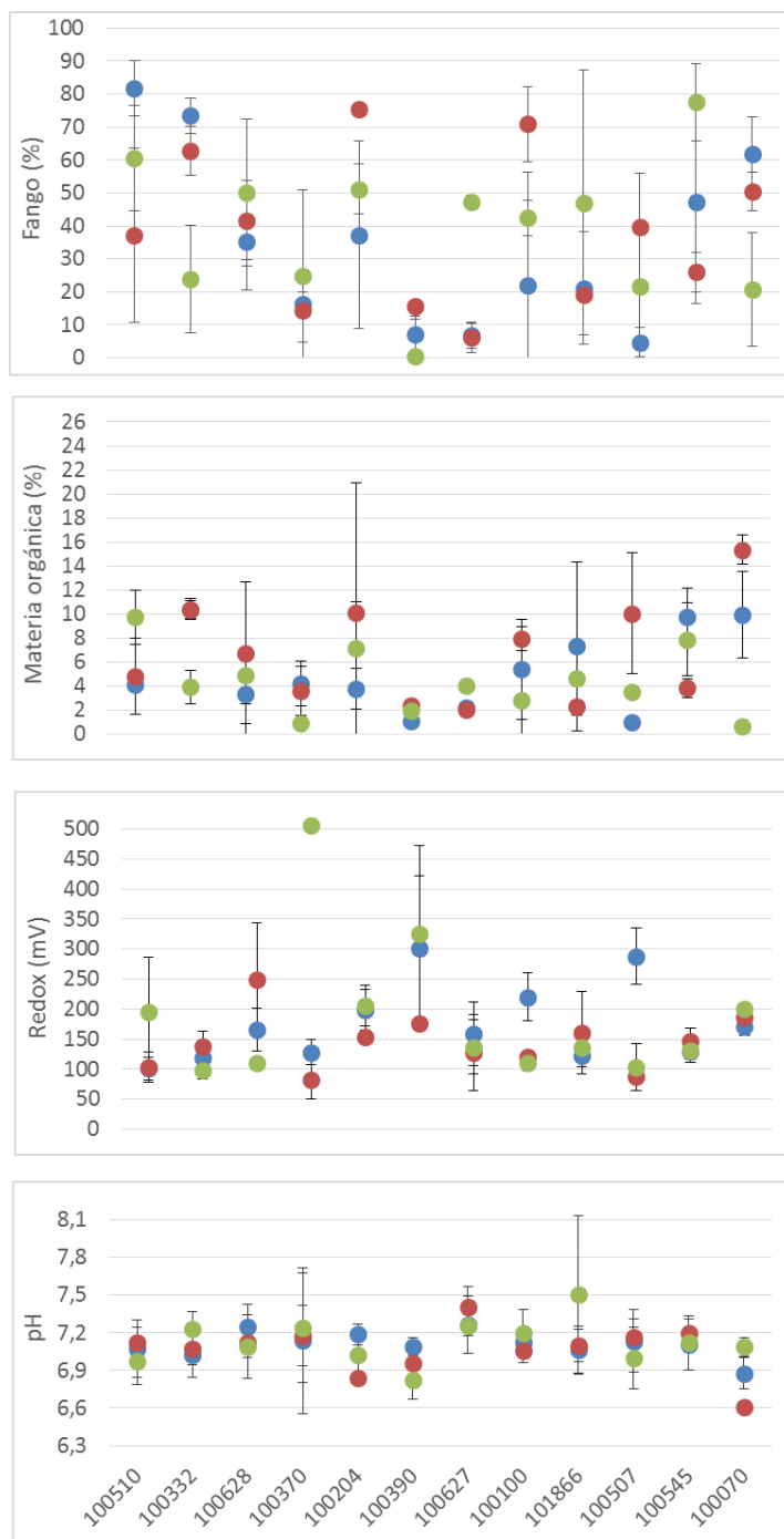
Figura 21. Lago Llanquihue: valores promedio y desviaci3n est3ndar de fango (%), materia org3nica (%), redox (mV) y pH en sedimentos para las diferentes estaciones de muestreo.
