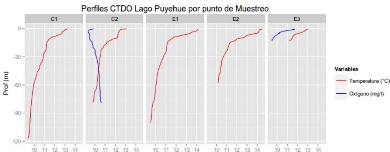
Figura 86. Perfiles físico-químicos (oxígeno en mg/L, y temperatura en °C) de la columna de agua de los centros analizados en el lago Puyehue.
