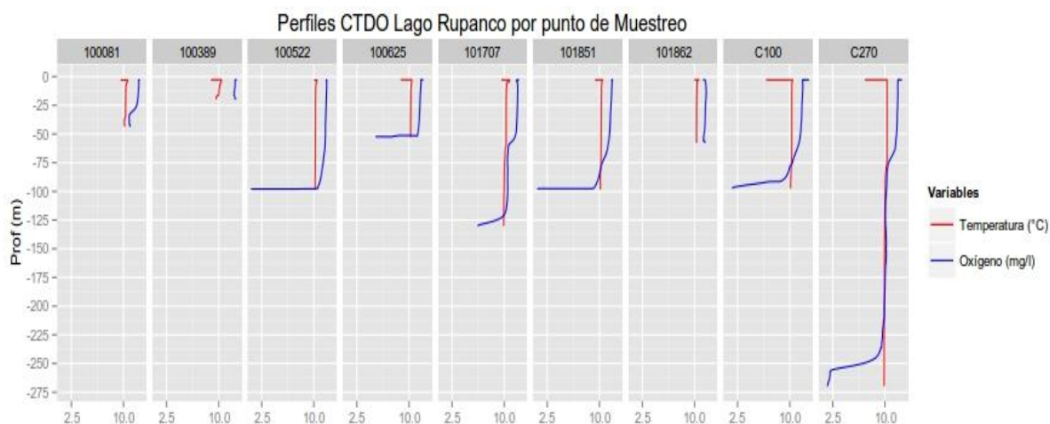
Figura 77. Perfiles fisico-qu3micos (ox3geno en mg/L y temperatura en °C) de la columna de agua en los centros analizados del lago Rupanco.
