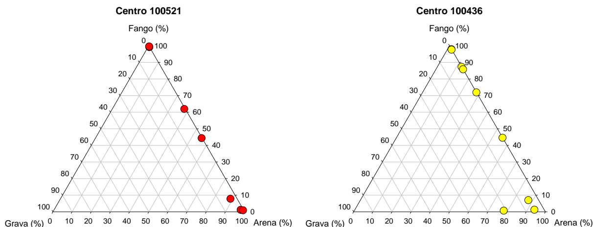
Figura 55. Lago Tarahuín: Fracciones texturales (% fango, % arena y % grava) representadas en un gráfico de triángulo para cada centro.
