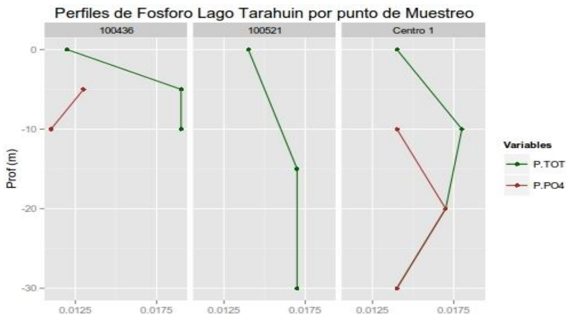
Figura 51. Perfiles de ortofosfato (P-PO 4 en mg/L) y fósforo total (PT en mg/L) en los centros analizados en el lago Tarahuín.
