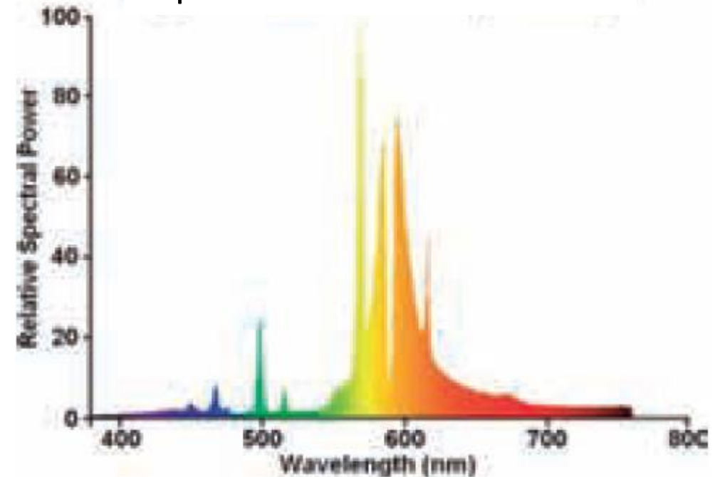
Espectro Sodio Alta Presión
